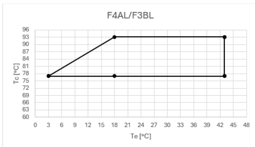
O nouă porțiune a limitelor de funcționare pentru compresorul F4AL/F3BL
