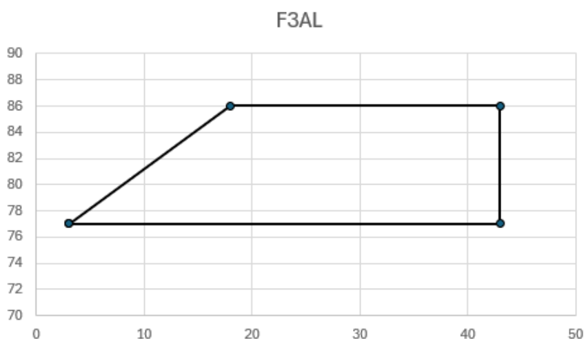
O nouă porțiune a limitelor de funcționare pentru compresorul F3AL
