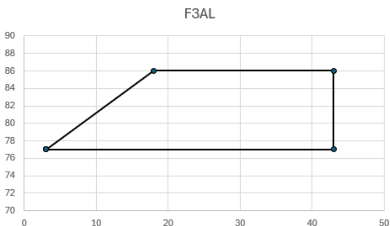
Nowa część limitów pracy sprężarki F3AL
