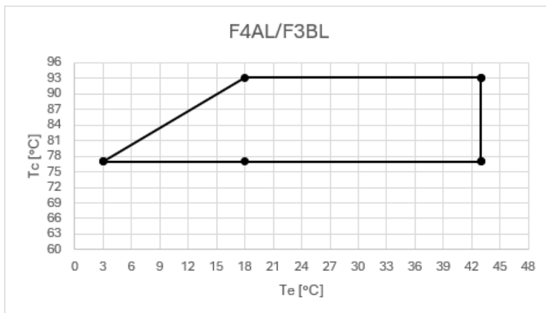
Nowa część limitów pracy sprężarki F4AL/F3BL
