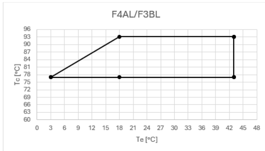
Neuer Hüllenteil für Kompressor F4AL/F3BL
