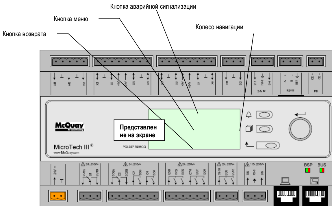
Рис. 7 Контроллер агрегата
