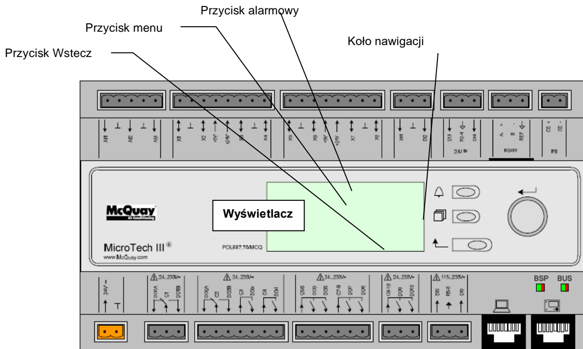
Rysunek 7, sterownik jednostki
