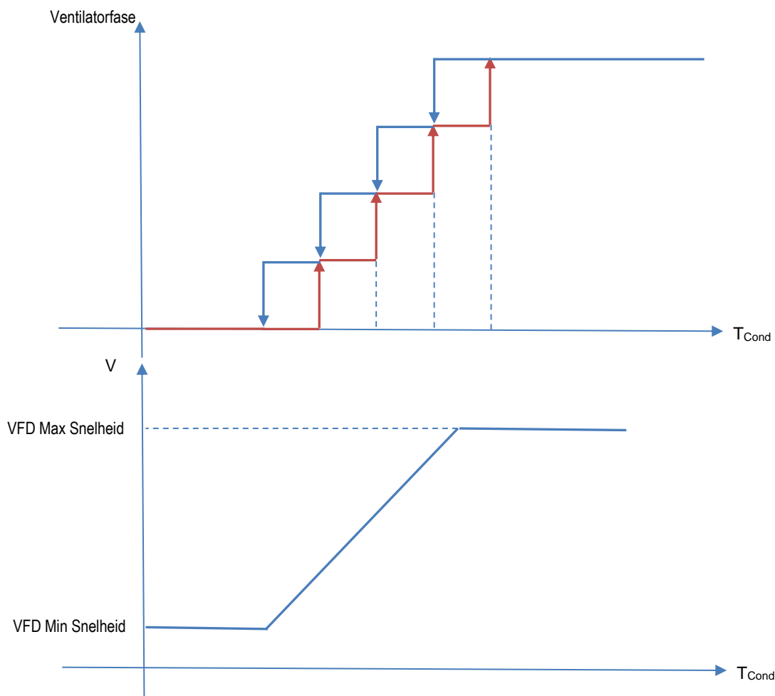
Afbeelding 6 – Watertemperatuur condensor
