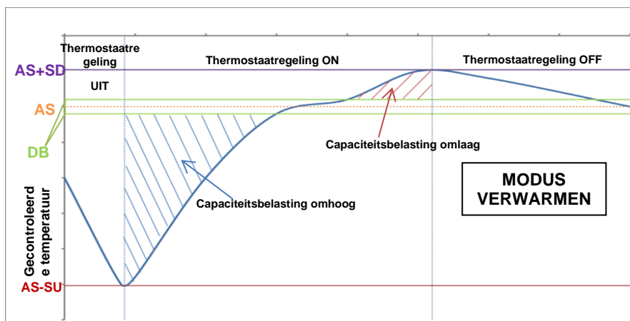
Afbeelding 5 – Instellingen thermostaatregeling
