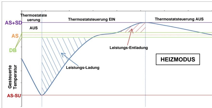
Abbildung 5 – Einstellungen Thermostatsteuerung
