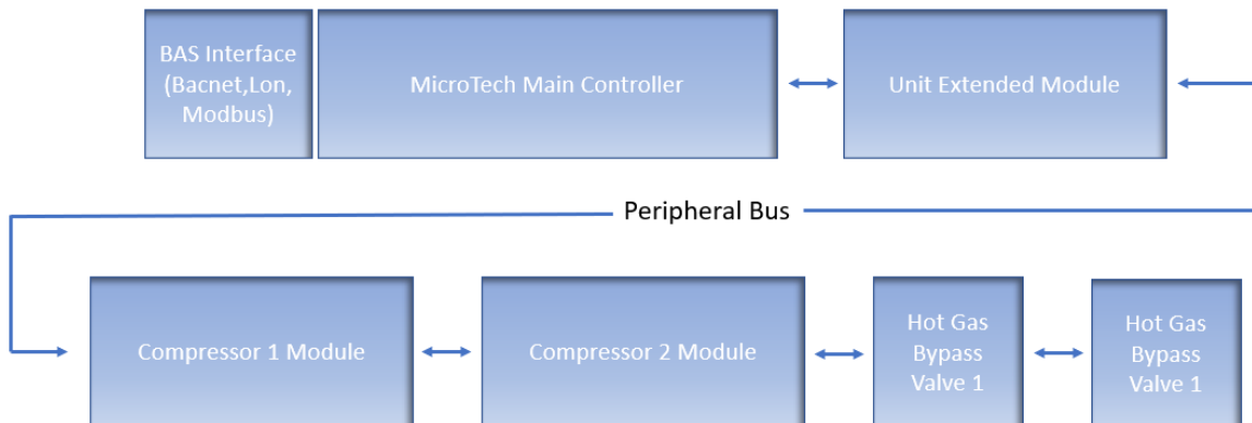
Abbildung 1 – Steuerungsarchitektur
