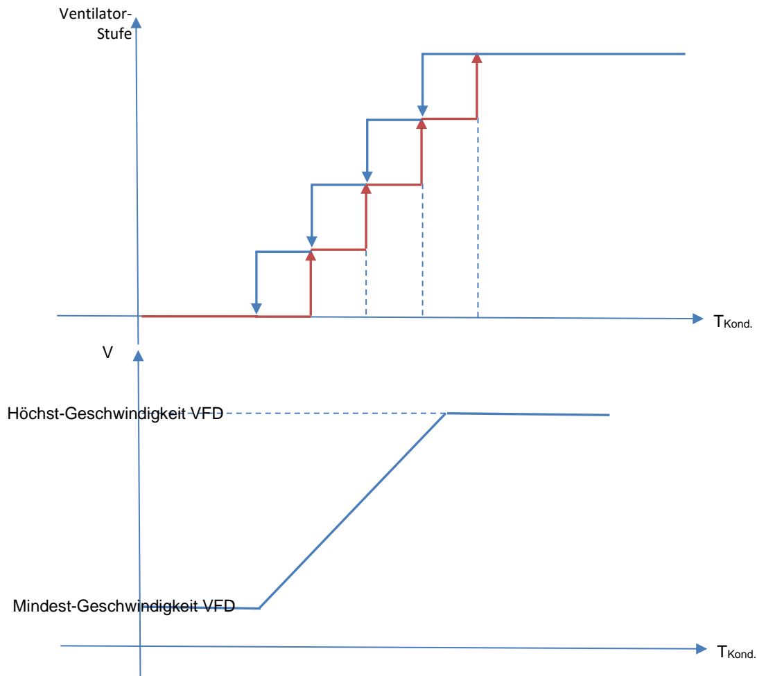
Abbildung 6 – Verflüssiger-Wassertemperatur
