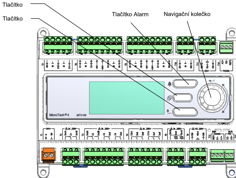
Obrázek 3 – Používání ovladače
