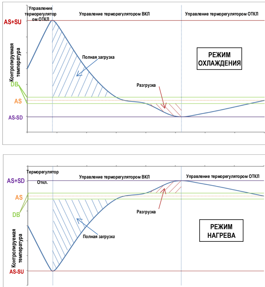
Рис. 5. Настройки терморегулятора
