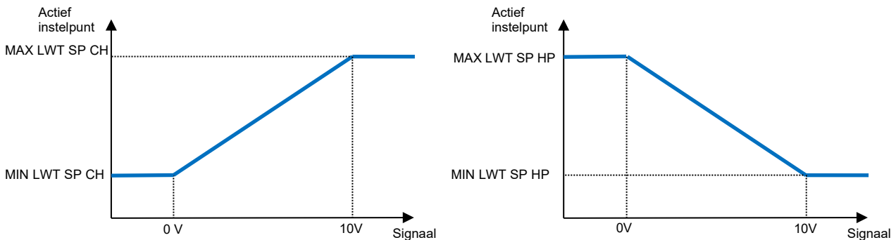
Grafiek 6 – 0-10V extern signaal versus Lwt-doel overschreven in koelmodus (links) en verwarmingsmodus (rechts)
