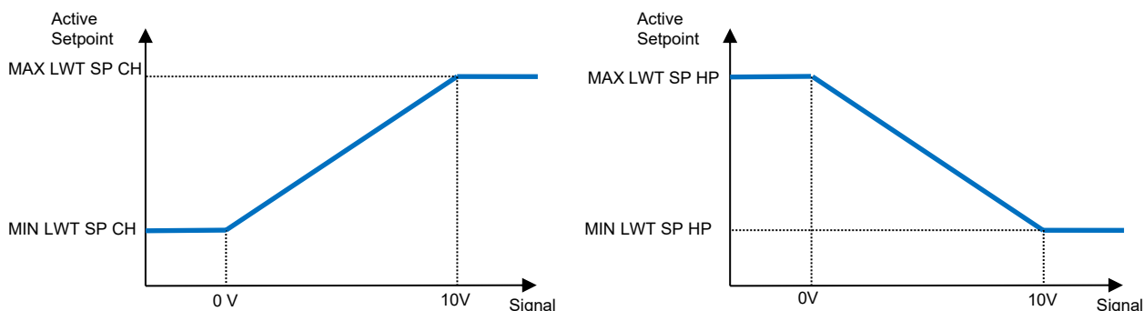
Grafikon 6 – 0-10V Külső jel vs Lwt Cél felülírva hűtési (bal) és fűtési módban (jobb)
