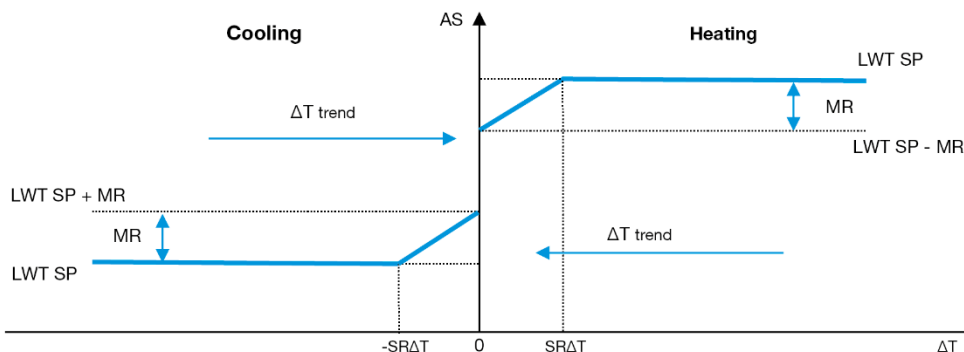
Grafiek 5 – Verdampers \Delta T tegen Actief Setpoint - Koelmodus (links) / Verwarmingsmodus (rechts)
