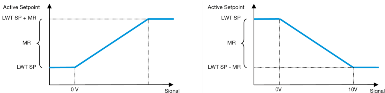
Graf 2 – Eksternt signal 0-10V vs Aktivt settpunkt - Kjølemodus(venstre)/ Oppvarmingsmodus(høyre)
