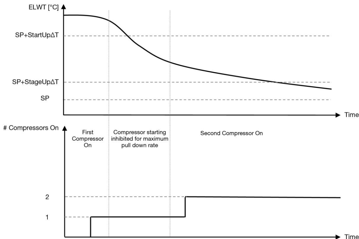
Graf 1 – Kompressorer oppstartsskvens - Kjølemodus
