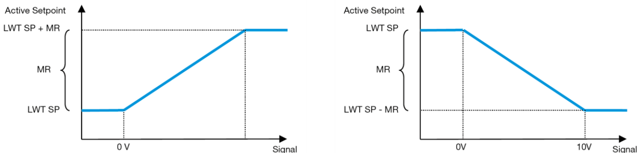
Grafiek 4 – Extern signaal 0-10V tegen Actief Setpoint - Modus Koelen (links)/ Modus Verwarmen (rechts)
