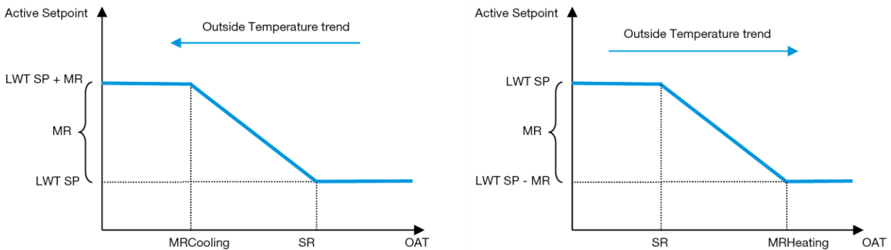
Grafiek 3 – Omgevingstemperatuur tegen Actief Setpoint - Modus Koelen (links) / Modus Verwarmen (rechts)
