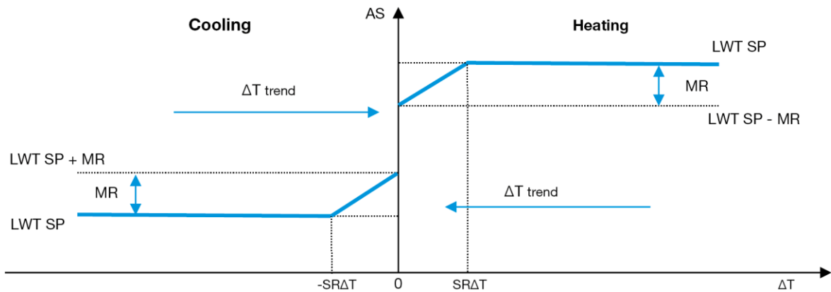
Grafiek 5 – Verdamer \Delta T tegen Actief Setpoint - Modus Koelen (links) / Modus Verwarmen (rechts)
