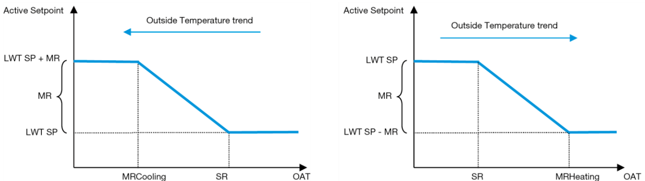
3. grafikon – Külső környezeti hőmérséklet vs Aktív beállítási pont - Hűtés mód (balra)/Fűtés mód (jobbra)
