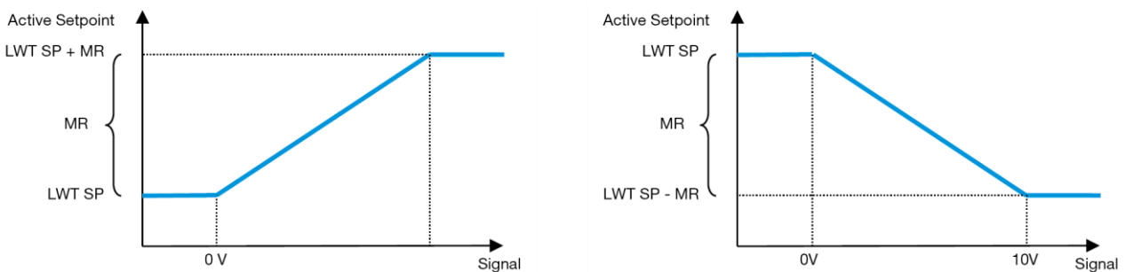
4. grafikon – Külső 0-10 V jel vs Aktív beállítási pont - Hűtés mód (balra) / Fűtés mód (jobbra)
