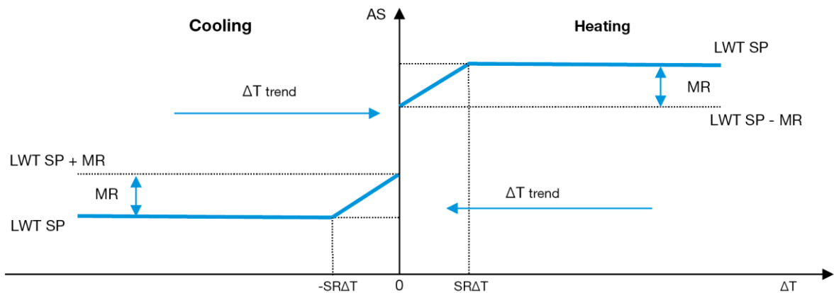
5. grafikon – Párol. ΔT vs Aktív beállítási pont - Hűtés mód (balra)/Fűtés mód (jobbra)
