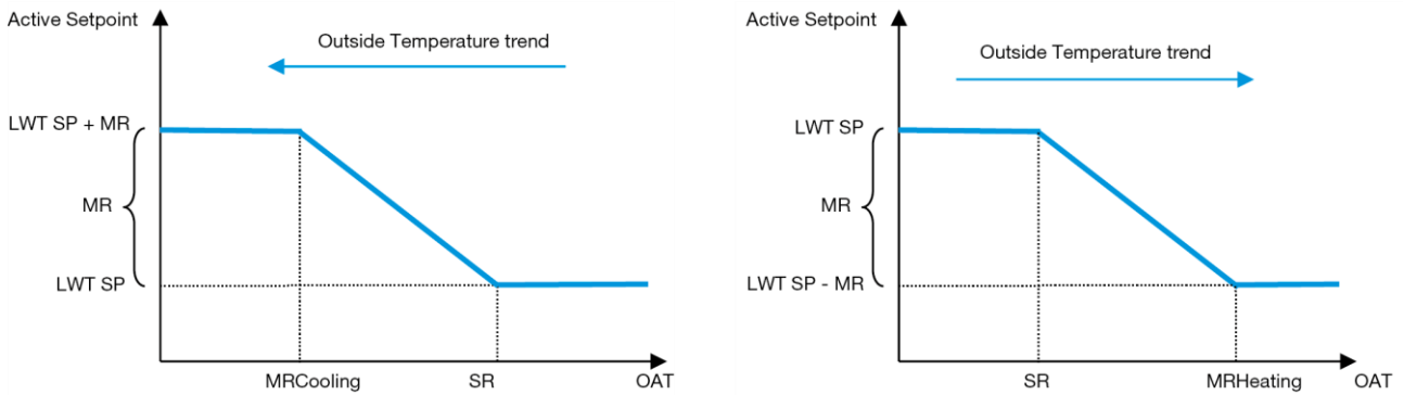
Γράφημα 3 – Εξωτερική θερμοκρασία περιβάλλοντος και Ενεργό Σημείο Ορισμού - Λειτουργία Ψύξης (αριστερά) / Λειτουργία Θέρμανσης (δεξιά)
