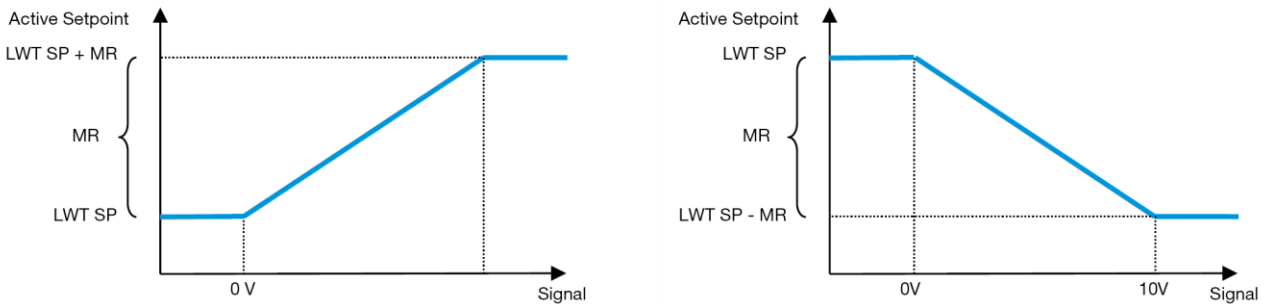
Γράφημα 4 – Εξωτερικό σήμα 0-10V και Ενεργό Σημείο Ρύθμισης - Λειτουργία Ψύξης (αριστερά) / Λειτουργία Θέρμανσης (δεξιά)
