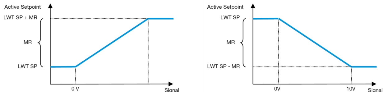
Grafic 4 – Semnalul extern 0-10 V față de valoarea de referință activă - modul Răcire (stânga)/modul Încălzire (dreapta)
