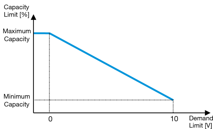
Γράφημα 2 – Περιορισμός ζήτησης[V] και Όριο απόδοσης[%]
