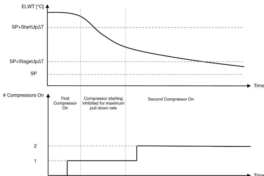
Γράφημα 1 – Ακολουθία εκκίνησης συμπιεστών - Λειτουργία ψύξης
