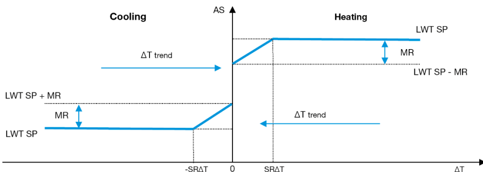
Γράφημα 5 – Έναρ ΔΤ (Διαφορά θερμοκρασίας για εξατμιστή) και Ενεργό Σημείο Ορισμού - Λειτουργία Ψύξης (αριστερά) / Λειτουργία Θέρμανσης (δεξιά)
