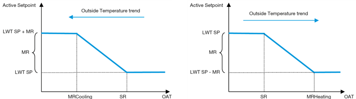
Graphique 3 – Température ambiante vs. Point de consigne actif - Mode Refroidissement (à gauche) / Mode Chauffage (à droite)
