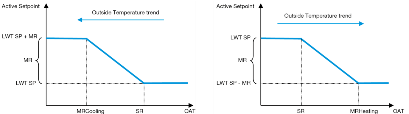
Diagramm 3 – Außenlufttemperatur gegenüber aktivem Sollwert – Kühlmodus (links)/Heizmodus (rechts)
