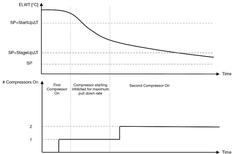
Diagramm 1 – Startsequenz der Verdichter - Kühlmodus
