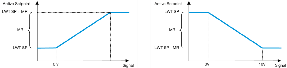
Diagram 4 – Externí signál 0-10 V vs Aktivní zadaná hodnota - Režim chlazení (vlevo) / Režim vytápění (vpravo)
