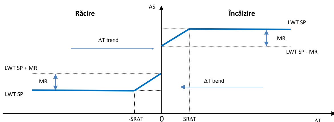
Grafic 4 Evap \Delta T față de valoarea de referință activă - modul Cooling (de răcire) (stânga) / modul Heating (de încălzire) (dreapta)
