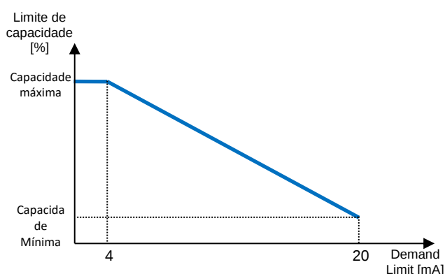
Gráfico 1 Limite exigido[mA] vs Limite de capacidade[%]
