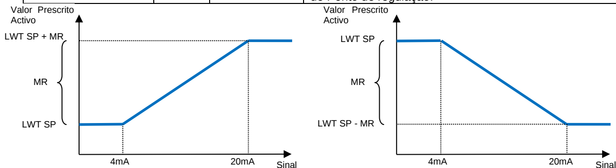
Gráfico 3 Sinal externo 4-20mA vs Ponto de regulação Ativo - Modo de arrefecimento (esquerda)/Modo de aquecimento (direita)
