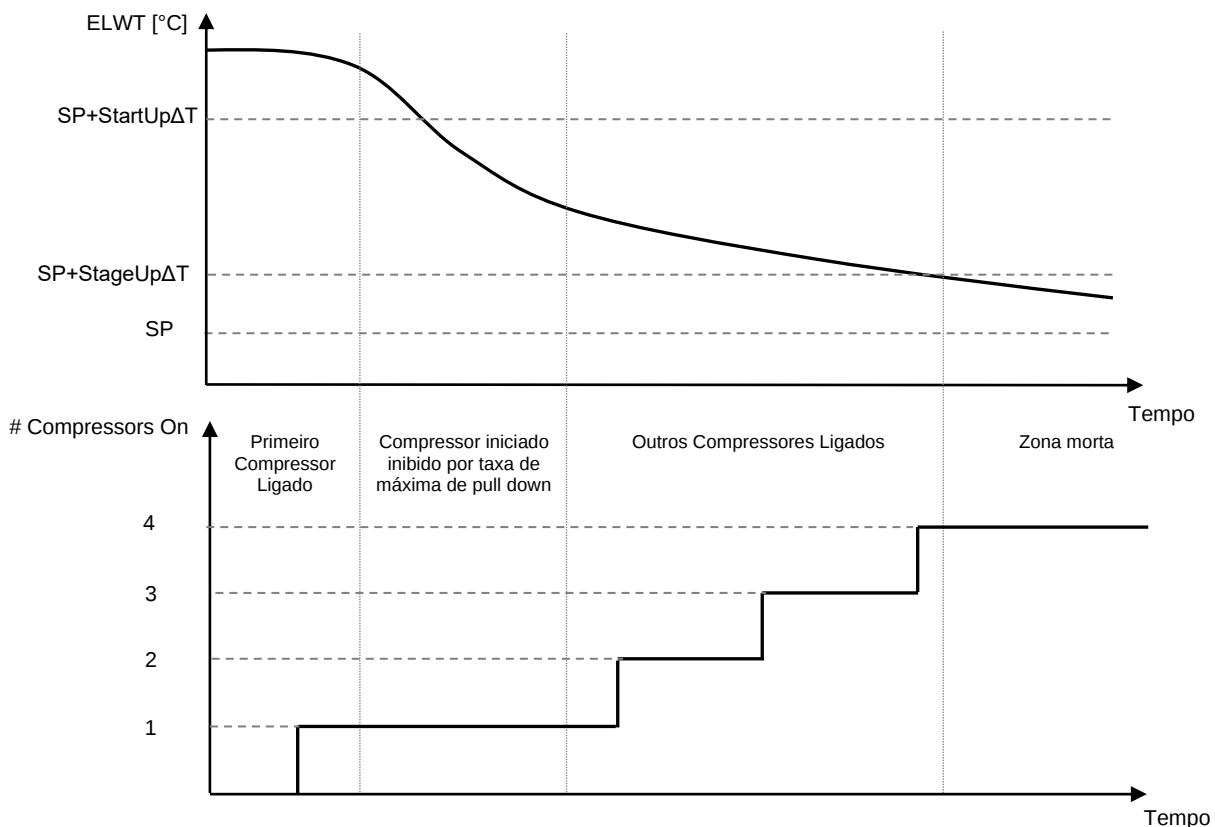
Sequência de start-up de compressores – Cool Mode
