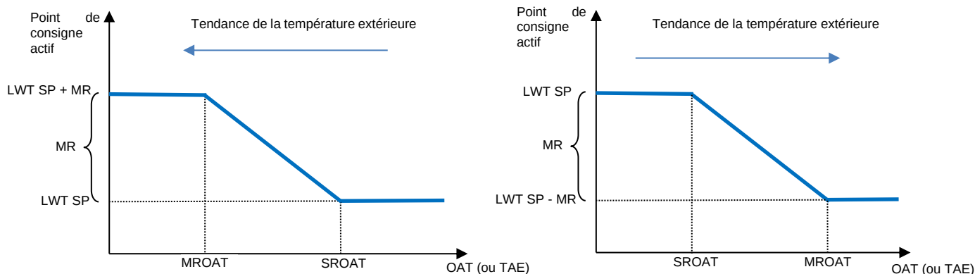
Graphique 2 Température ambiante vs. Point de consigne actif - Mode Refroidissement (à gauche) / Mode Chauffage (à droite)
