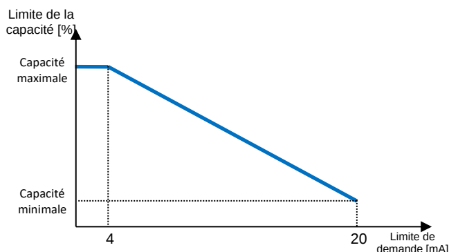
Graphique 1 Limite de demande [mA] vs Limite de capacité [%]
