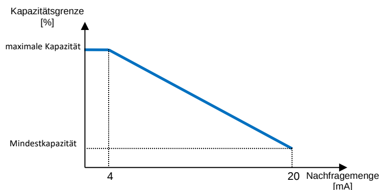
Graph 1 Bedarfsgrenze [mA] gegenüber Kapazitätsgrenze [%]
