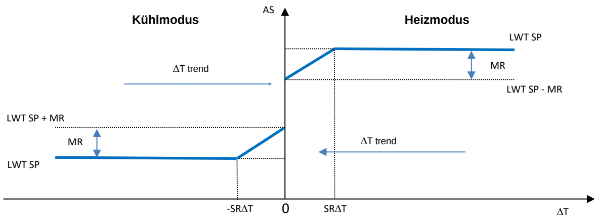
Graph 4 Verdampfer- \Delta T gegenüber aktivem Sollwert - Kühlmodus (links)/Heizmodus (rechts)
