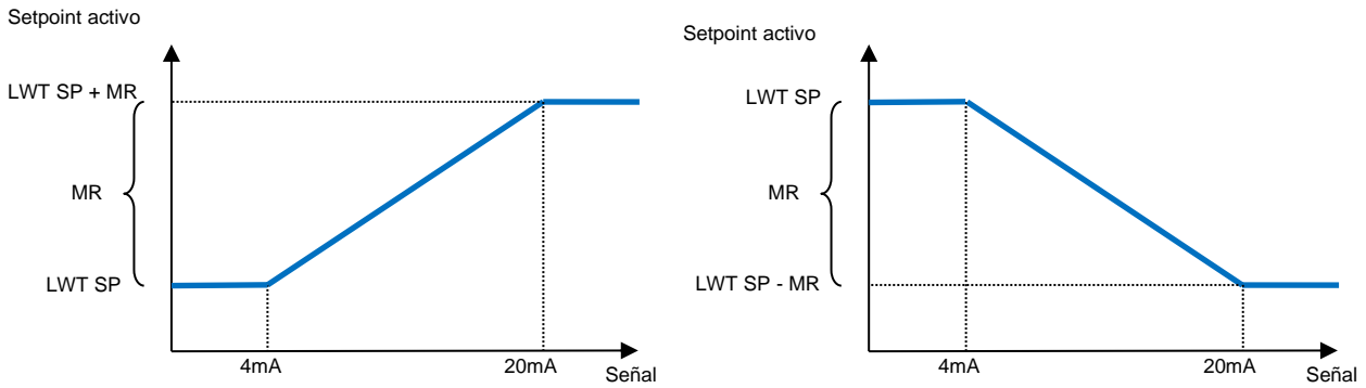
Gráfico 3 External Signal de 4-20mA vs Active Setpoint - Modo de enfriamiento (izquierda)/ Modo de calentamiento (derecha)
