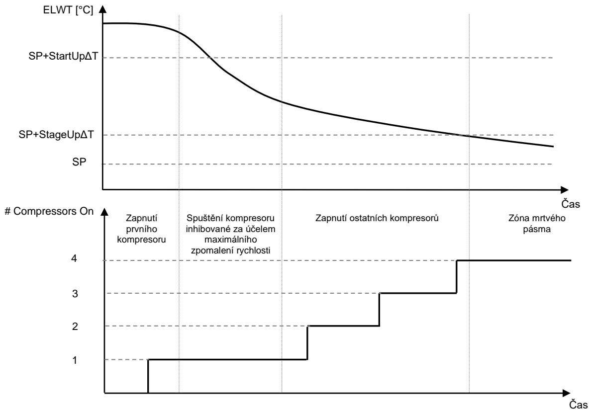
Sekvence spuštění kompresorů - Režim chlazení
