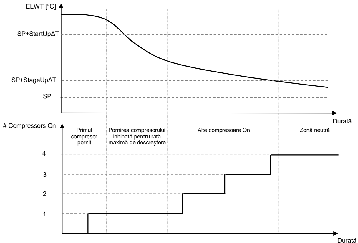
Secvența de pornire compresoare – Cool Mode
