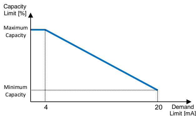
Grafic 1 Demand Limit (Limita de solicitare) [mA] vs Capacity Limit (Limita de capacitate) [%]
