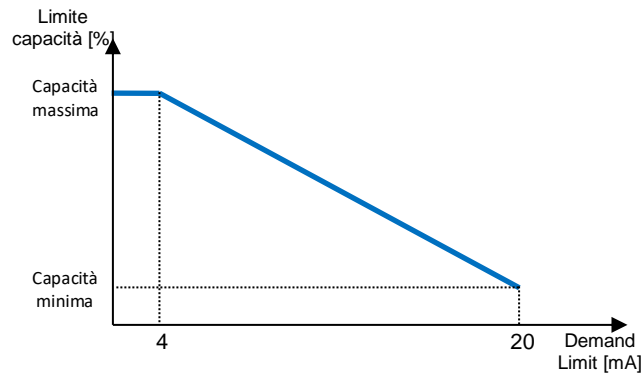
Gráfico 1 Limite Domanda [mA] vs Limite di Capacità [%]
