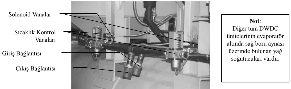
Şekil 12, Yağ Soğutucusu Bağlantıları, DWDC 100/126, 16 Foot Kabuk
