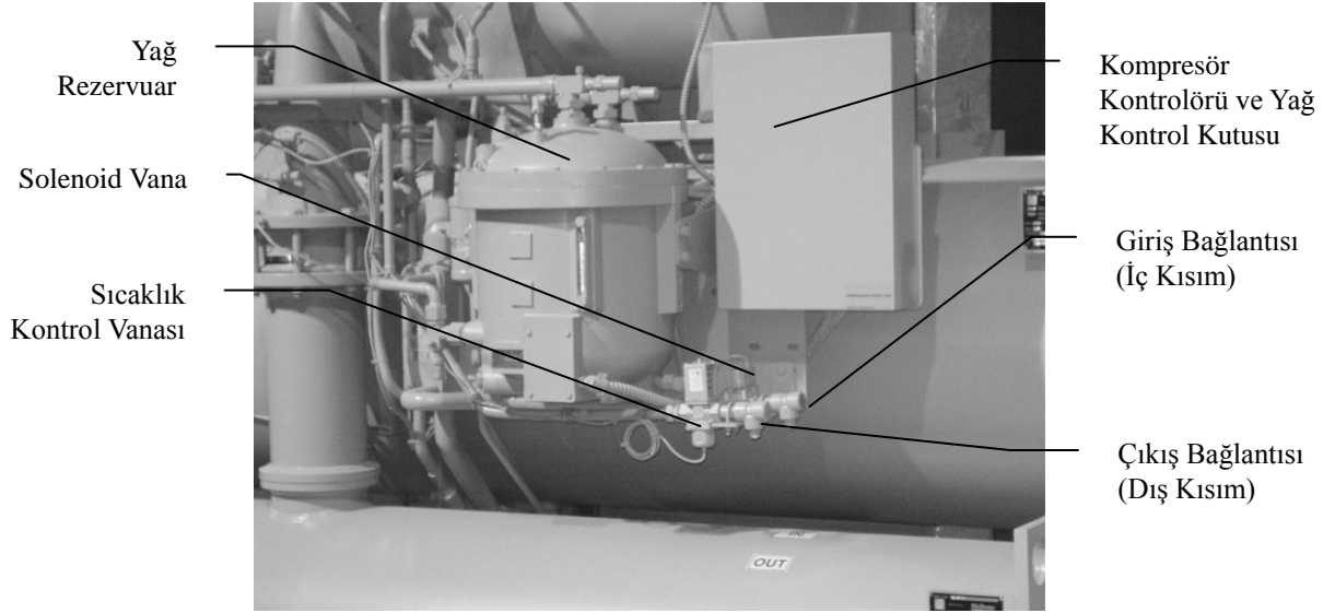
Şehir 11, Yağ Soğutucusu Bağlantıları, DWSC/DHSC Üniteleri
