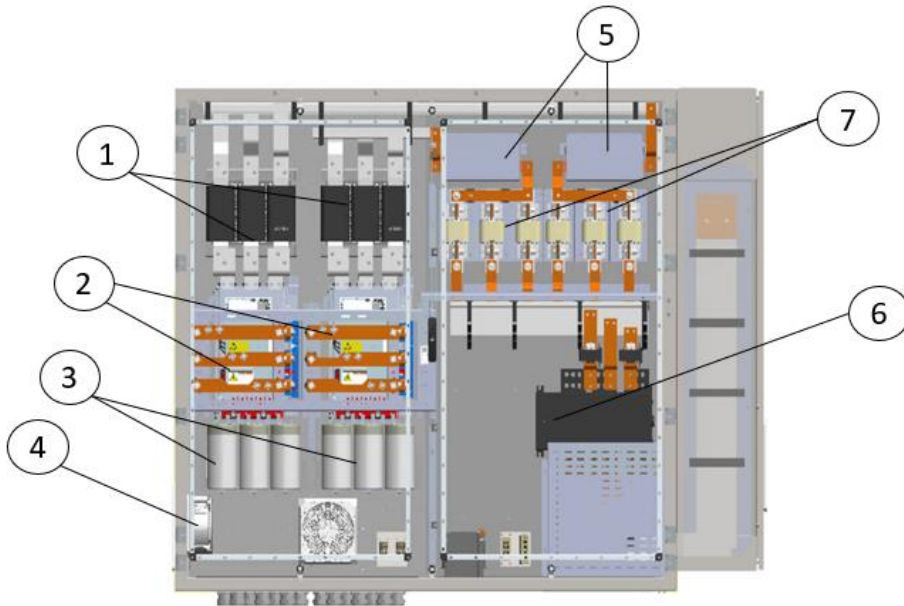
Рис. ° 24. Компоненты (двухконтурной) панели инвертора
