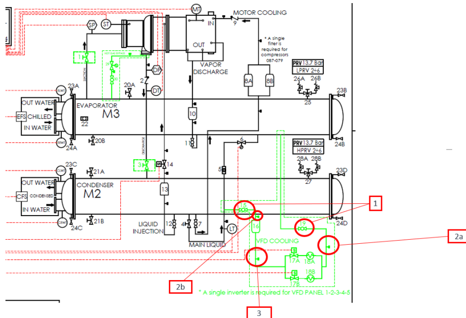
Fig. 23 - Diagrama de la unidad con detalle de la línea de refrigeración del inverser
