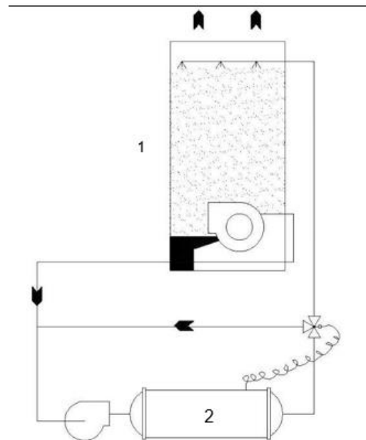
Fig. 6 - Esquema para el control de la condensación con torre de evaporación
