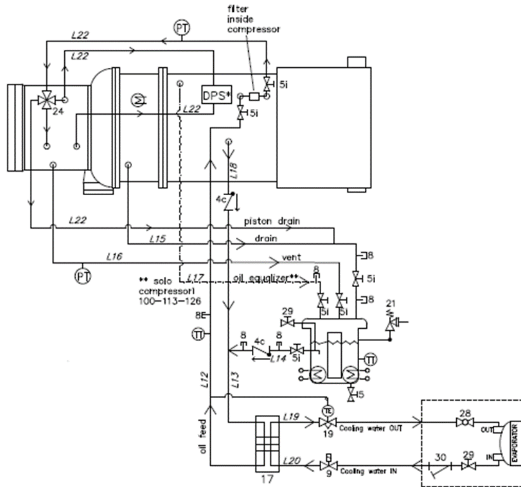
Fig. 1 - Circuito de aceite típico
