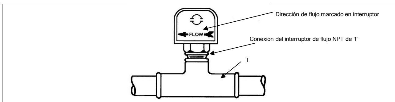
Fig. 8 - Montaje del interruptor de flujo
