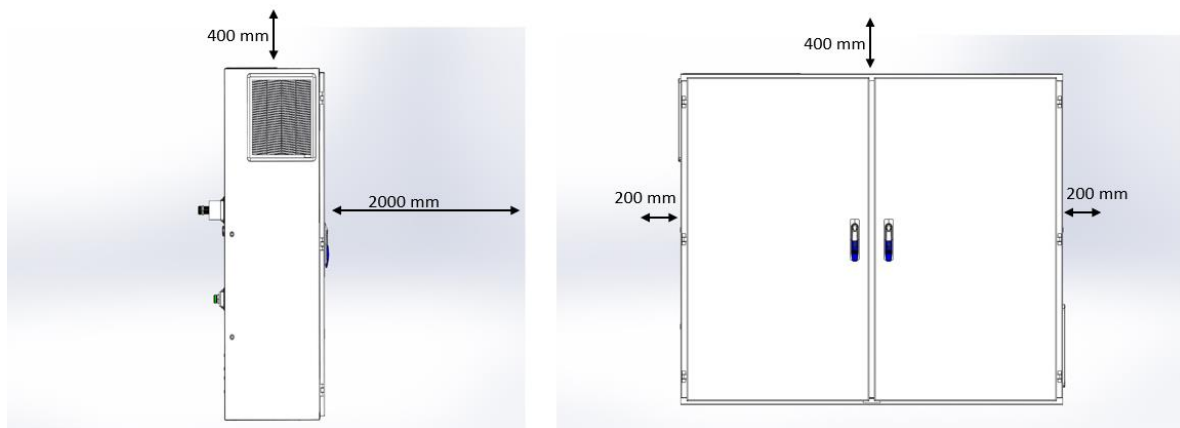
Fig. 16 - Requisitos de espacio mínimo para VFD
