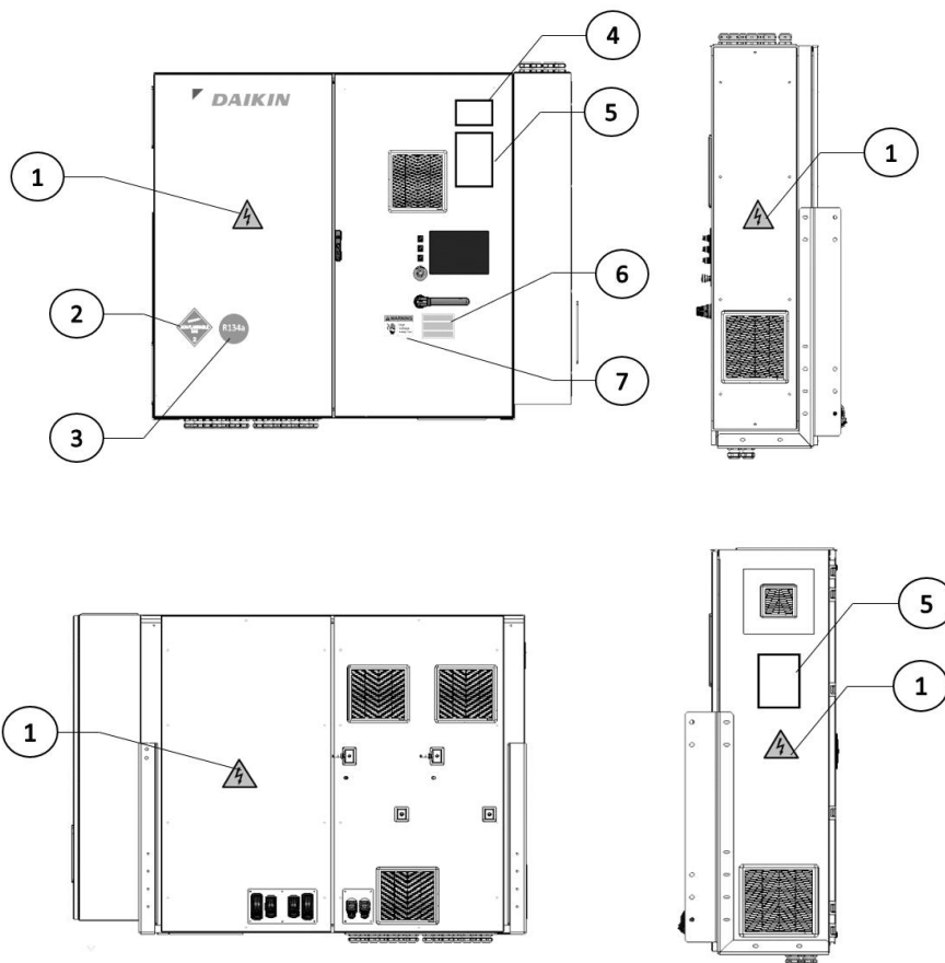
Fig. 2 - Descripción de las etiquetas aplicadas al panel eléctrico
