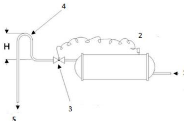
Fig. 7 - Esquema para el control de la condensación con agua de pozo
