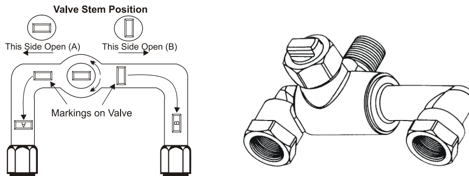
Fig. 12 - Válvula de 3 vías del condensador
