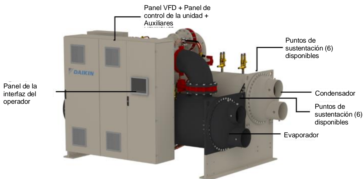
Fig. 5 - Disposición de los componentes principales de la serie DWSC
