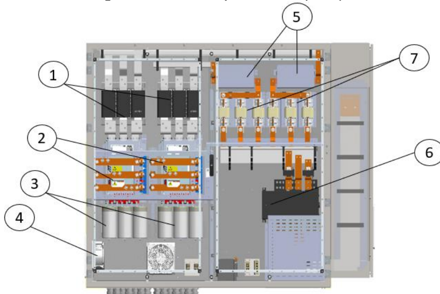
Fig. 21 - Elementos del panel inverter (doble)
