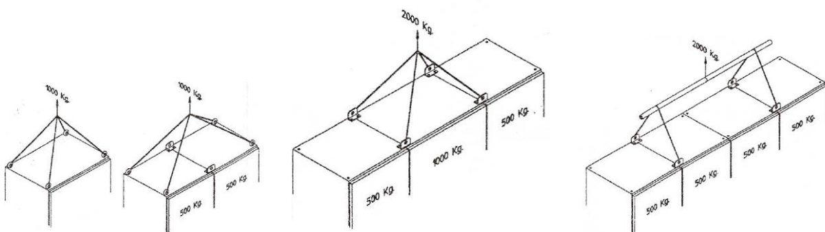
Fig. 15 - Elevación del VFD
