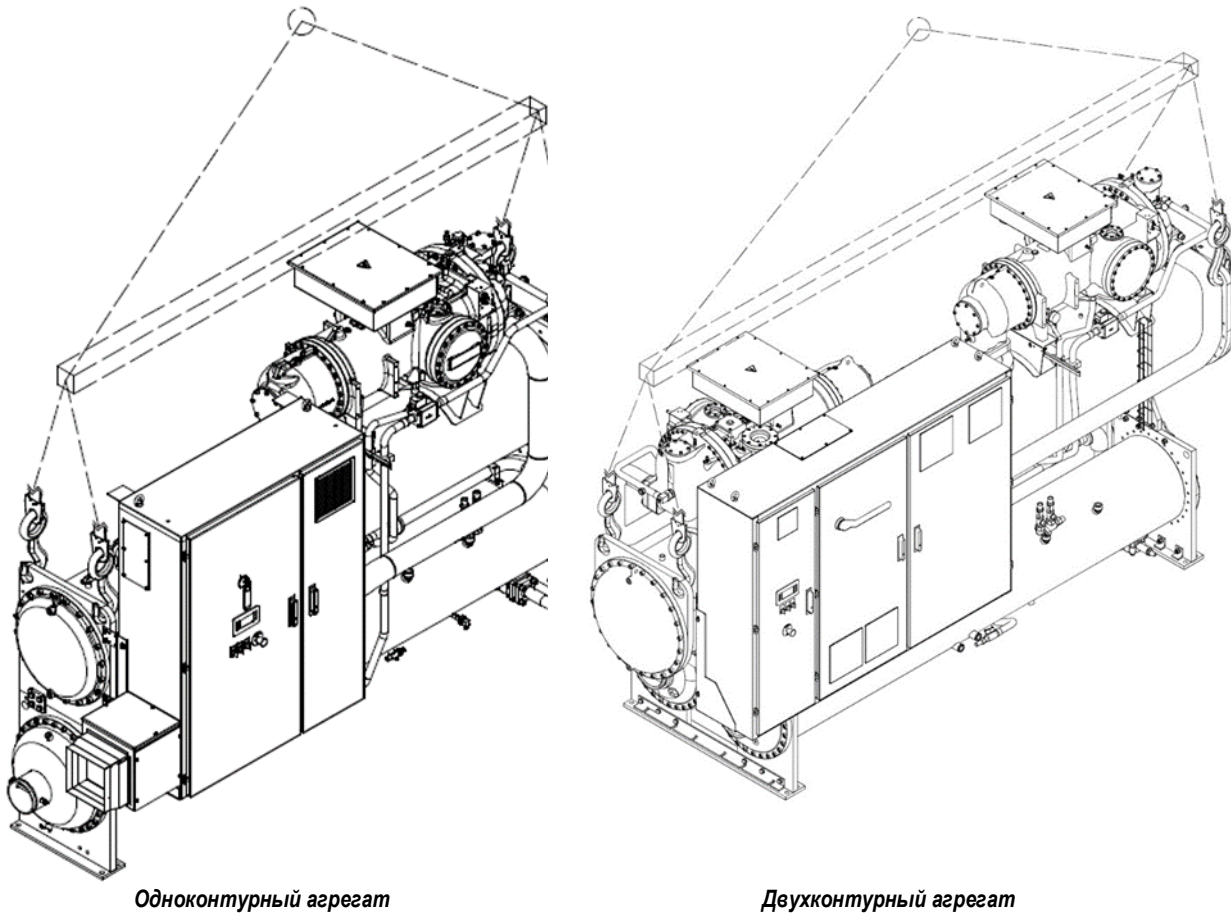
Рис. 3. Инструкции по подъему
