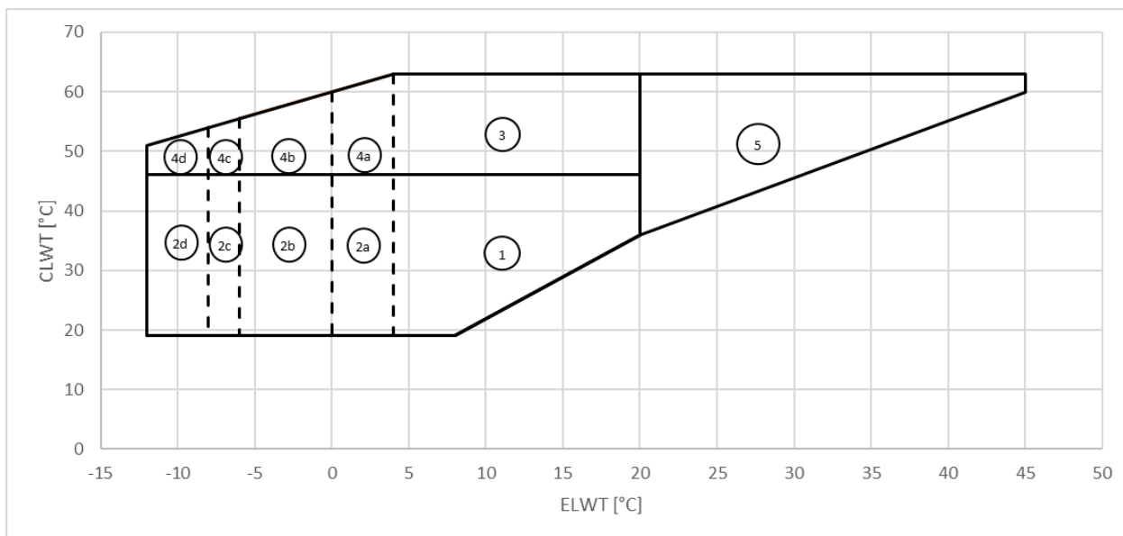
Рис. 5. Рабочий диапазон EWWD_VZ_SS
