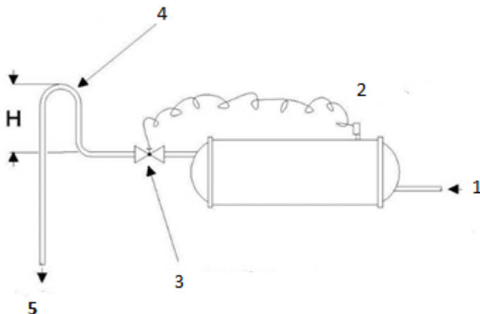
Рис. 12. Схема управления конденсацией при использовании артезианской воды
