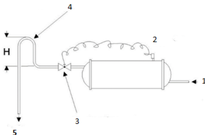
Figură 12 - Schema de control a condensatorului cu apă de fântână
