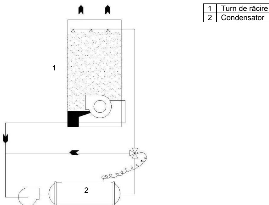
Figură 11 - Schema de control a condensatorului cu turn de răcire
