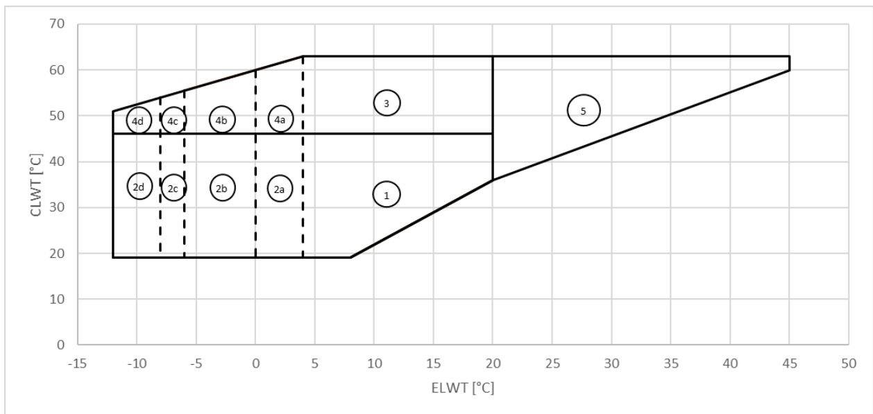
Figură 5 - Îneliş EWWD_VZ_SS
