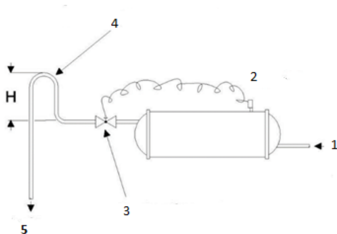
Схема12 - Схема за контрол на кондензацията с вода от кладенец
