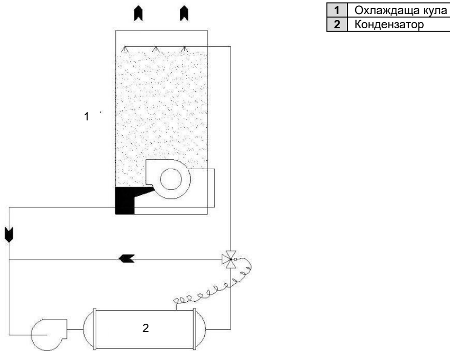
Схема11 - Схема за управление на кондензатора с охладителна кула
