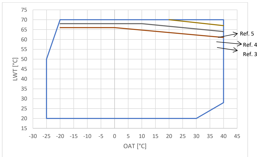
Figura 2 - Límites operativos en EWYE-CZ
