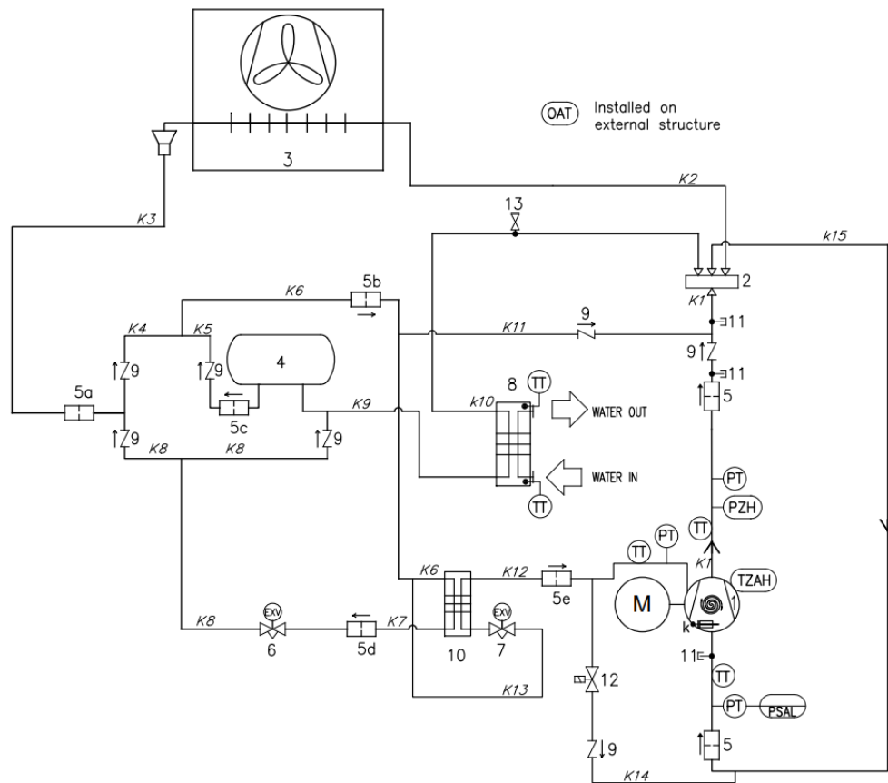
Εικόνα 16 - Διάγραμμα κυκλώματος ψυκτικού μέσου (P&ID) για μονάδα ΜΟΝΟΥ κυκλώματος ΕWYE~CZ
