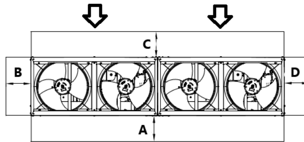
Εικόνα 8 – ΔΙΠΛΗ μονάδα
