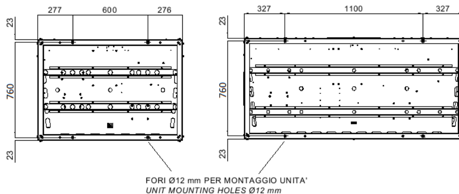
Рис. 7 – Расположение монтажных отверстий (вид снизу)
