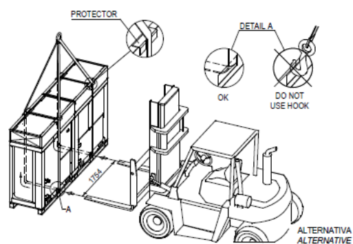
Рис. 3 – Подъем агрегата с одним контуром
