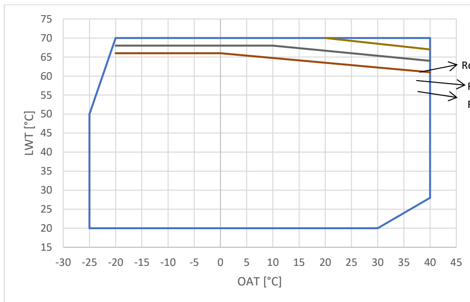
Рис. 2 - Эксплуатационные пределы для EWYE-CZ
