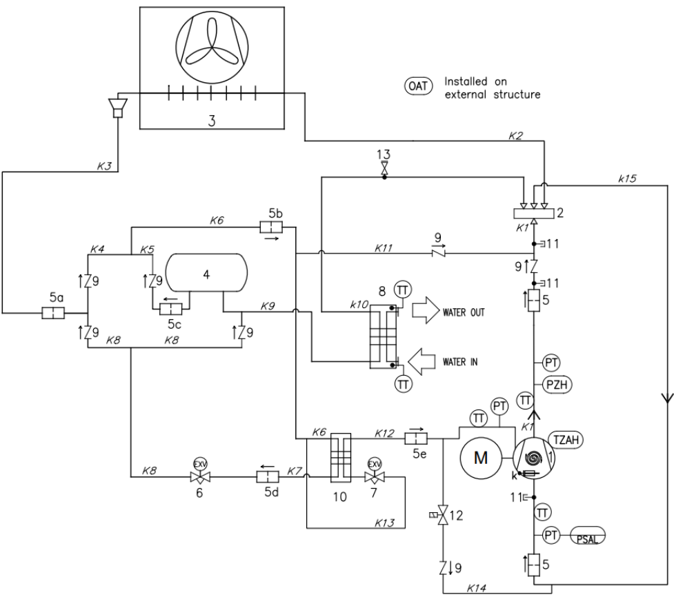
Рис. 15 - Схема контура хладагента (СТИКИП) для контура агрегата с одним контуром EWYE-CZ
