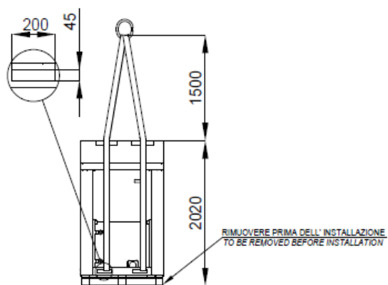
Рис. 3 – Подъем агрегата с одним контуром
