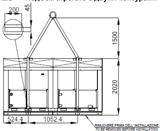
Рис. 4 – Подъем агрегата с двумя контурами
