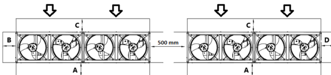
Рис. 9 – Агрегаты, установленные рядом друг с другом вдоль коротких сторон, B или D
