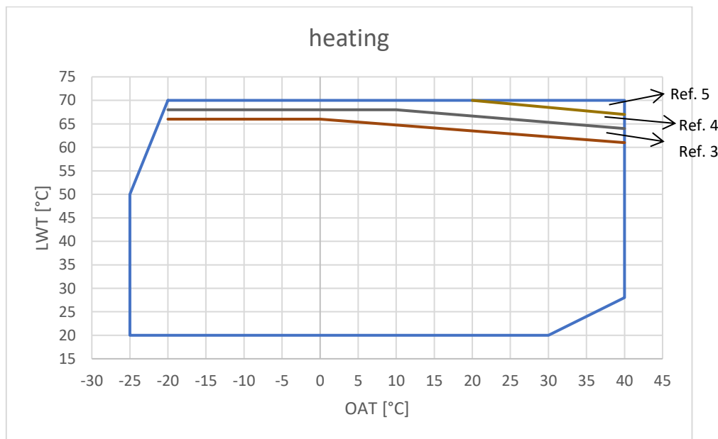
Figura 2 - Limiti operativi EWYE-CZ in modalità riscaldamento
