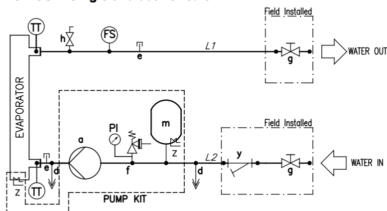
Figura 12 –Schema idraulico
