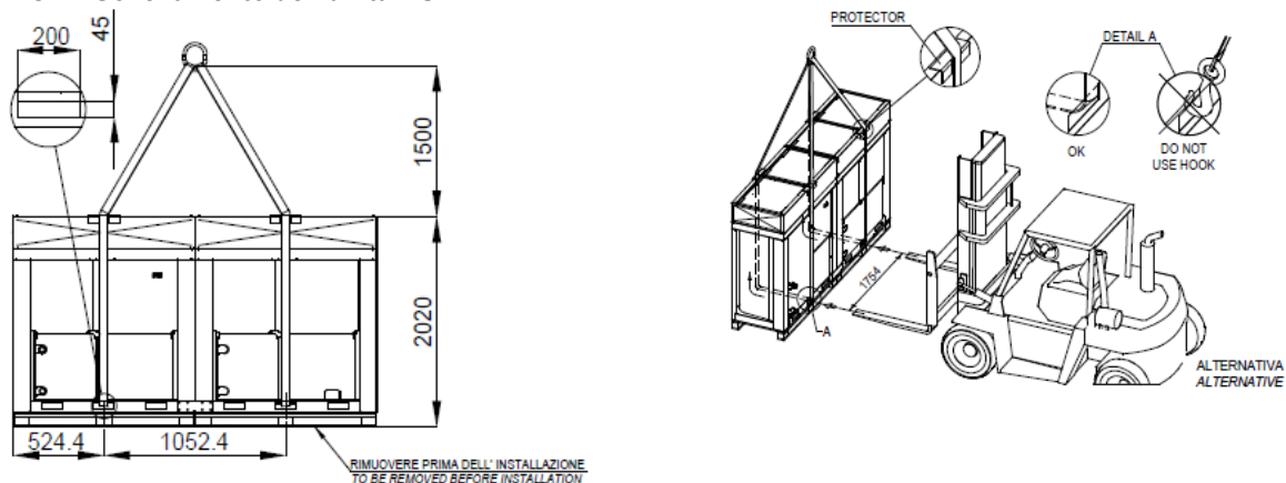
Figura 4 – Sollevamento unitàDUAL
