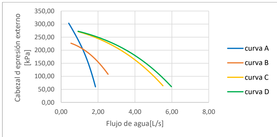
Figura 14 - Presión externa de bomba de elevación baja
