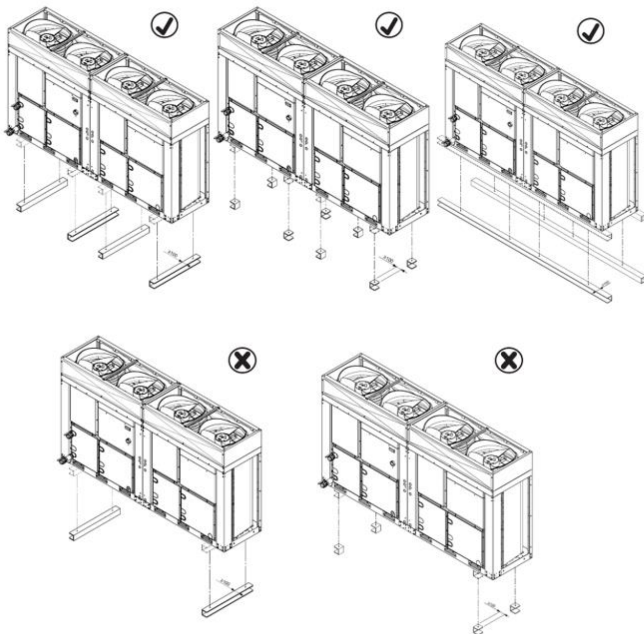
Εικόνα 6 – Τοποθέτηση ΔΙΠΛΗΣ μονάδας
