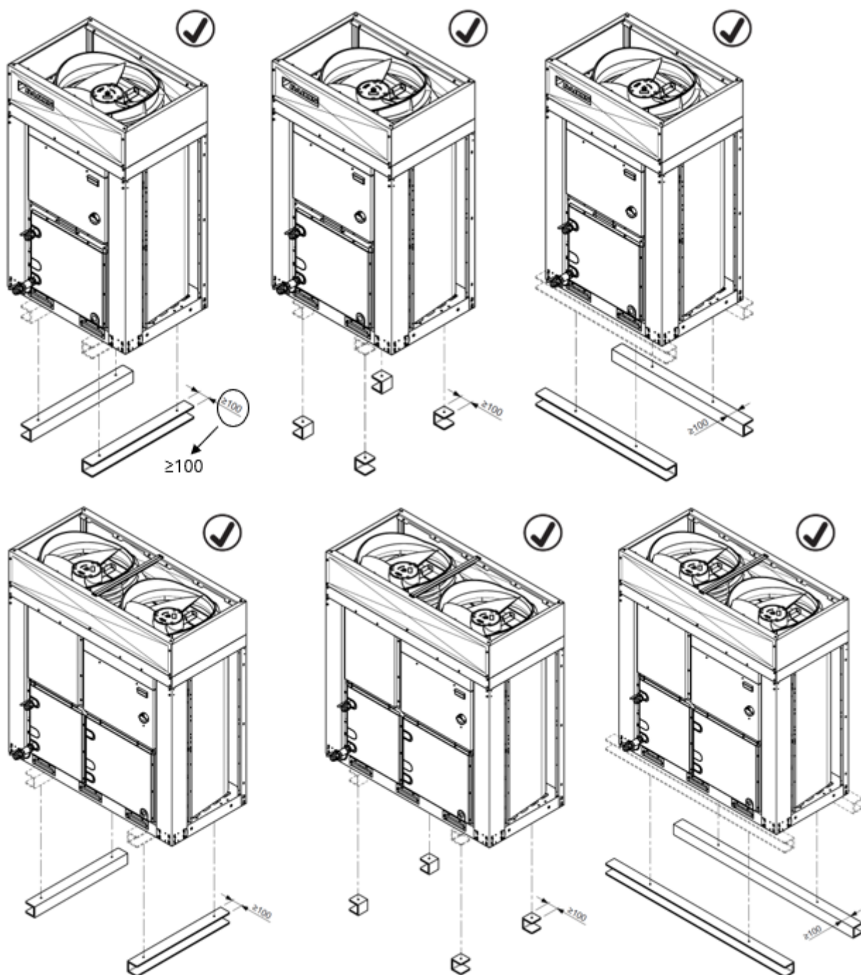
Εικόνα 5 – Τοποθέτηση ΜΟΝΗΣ μονάδας
