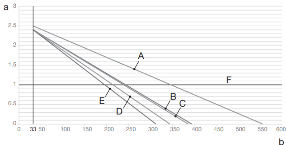
Εικόνα 15 - Αρχική πίεση δοχείου διαστολής με βάση τον μέγιστο όγκο νερού
