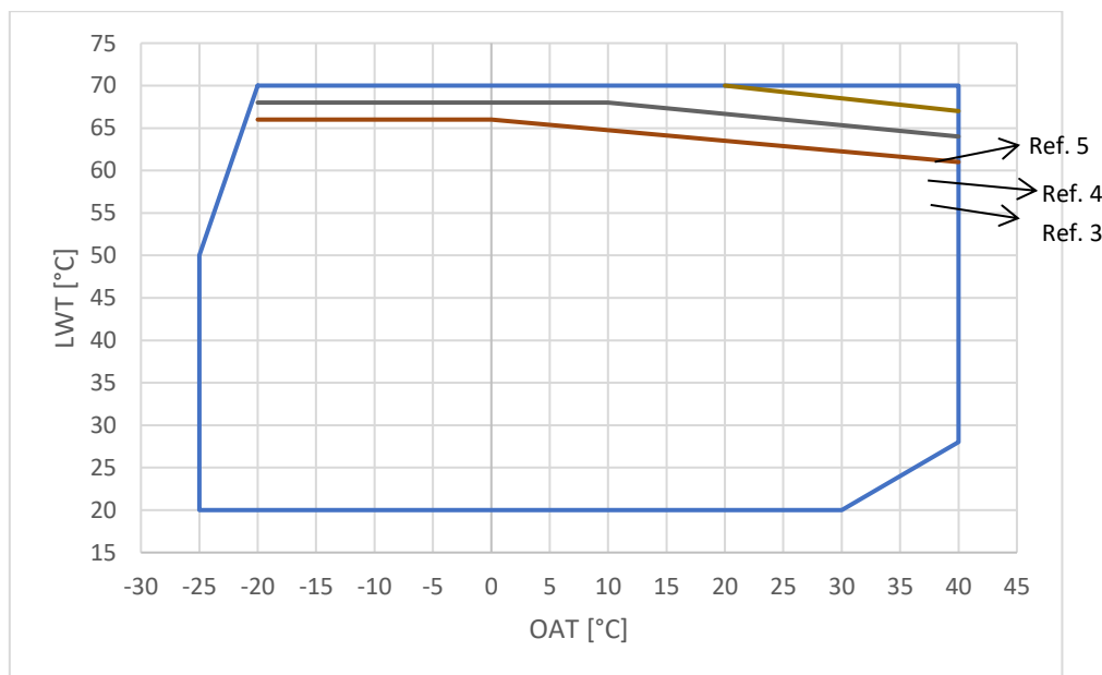
Εικόνα 2 - Όρια λειτουργίας στο EWYE-CZ
