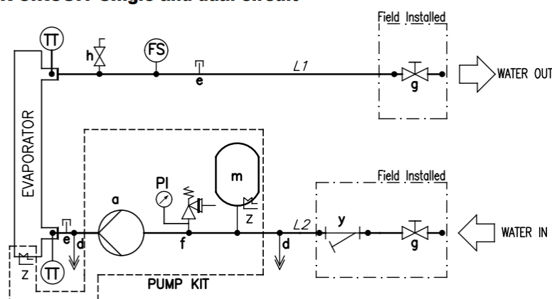
Εικόνα 12 – Υδραυλικό διάγραμμα
