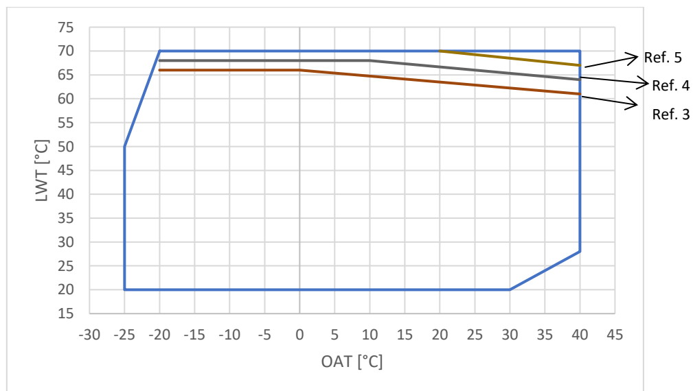
Abbildung 2 - Betriebsgrenzen für EWYE-CZ (Heizen)
