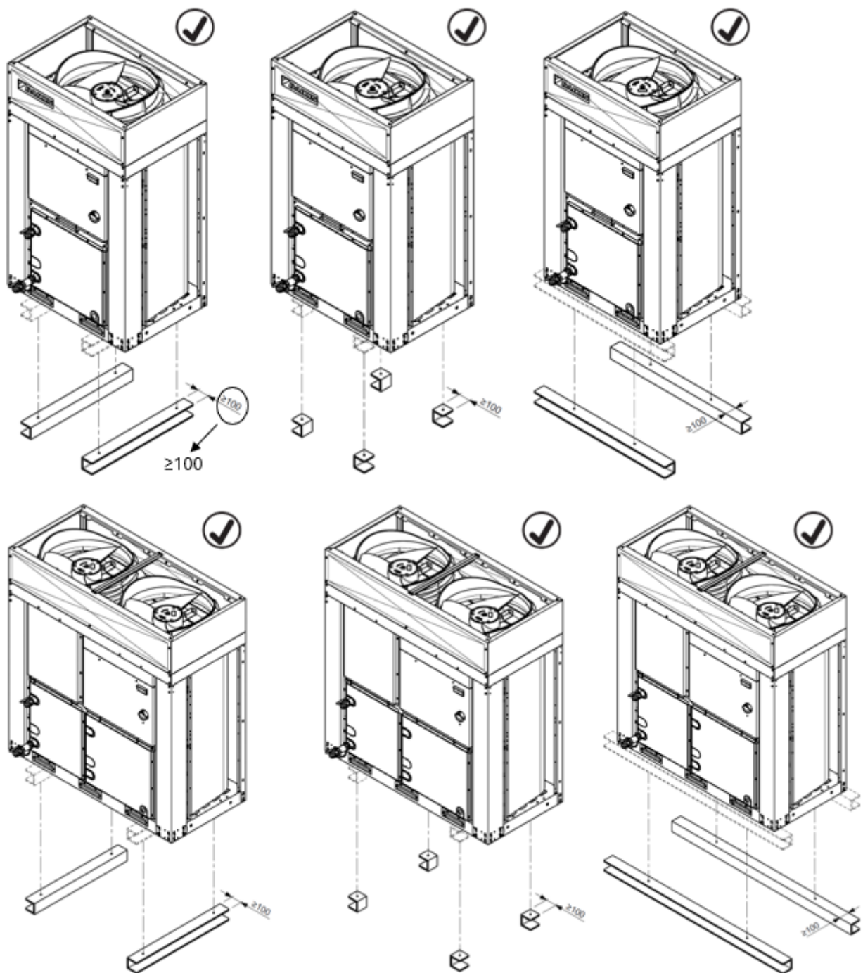
Abbildung 5 – Positionierung MONO-Gerät
