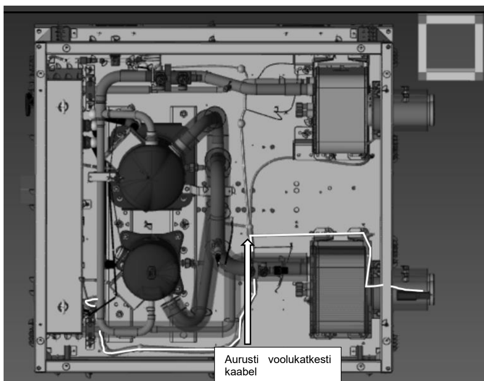
Joonis. 13 – Aurusti voolulüliti kaablite marsruut
