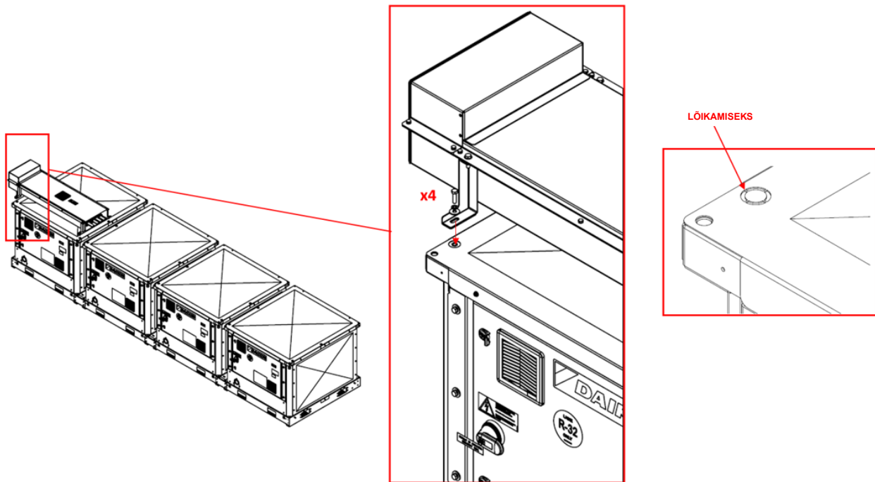
Joonis. 52 – Voolusiinisüsteemi kinnitamine seadme külge
