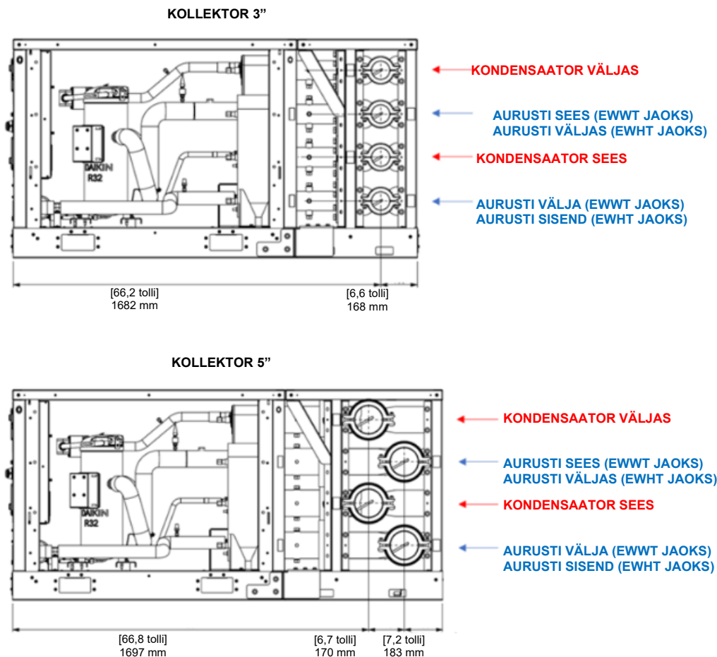
Joonis. 27 – Veekollektori suurused
