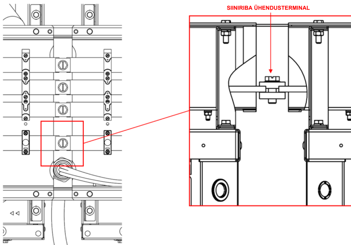
Joonis. 54 – Üksikasjad voolusiinimoodulite ühendamise kohta
