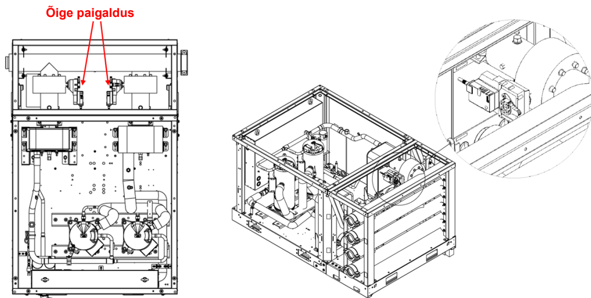
Joonis. 31 – Ventili täituri paigaldusjuhised
