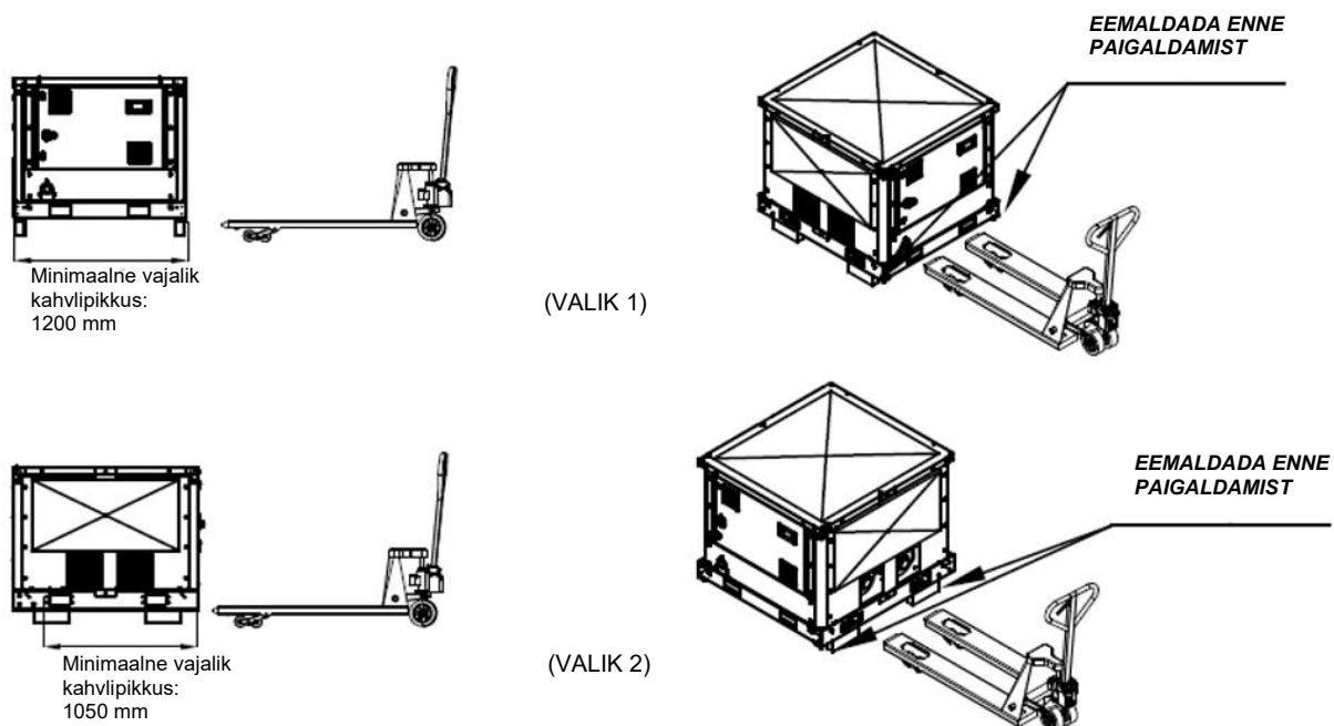
Joonis. 48 – Pumbamoodulit saab käsitseda alusekäruga, kui selle alla on paigaldatud puidust vahetükid
