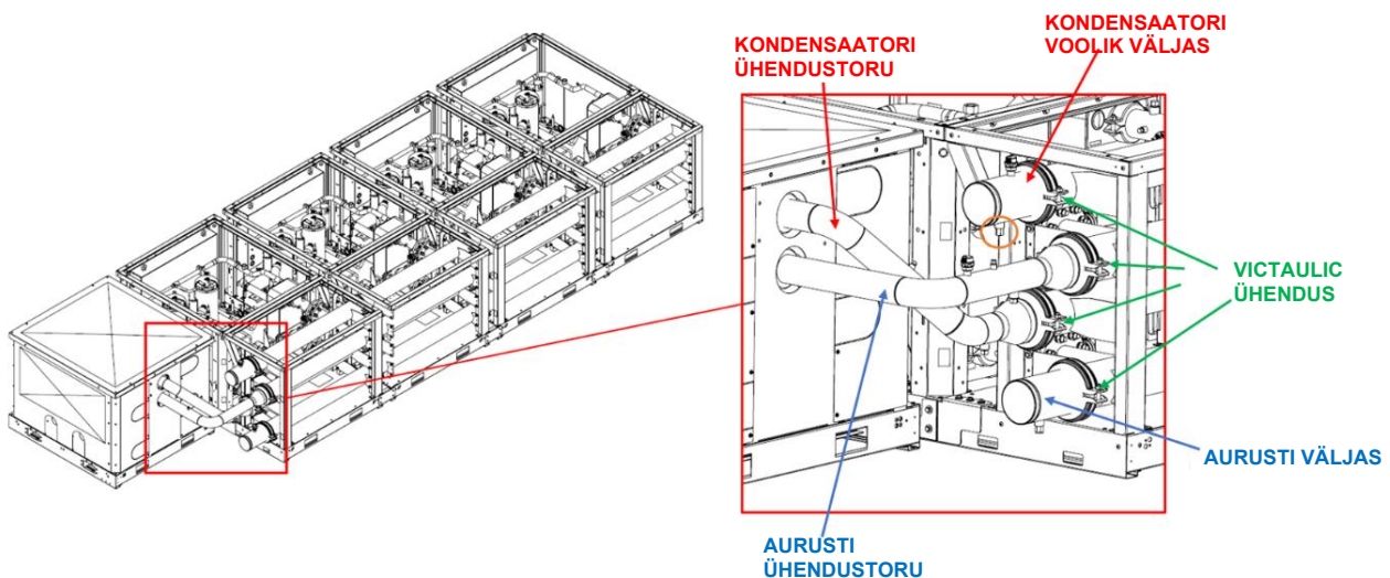
Joonis. 43 – Pumbamooduli paigaldamine – torustiku detailid
