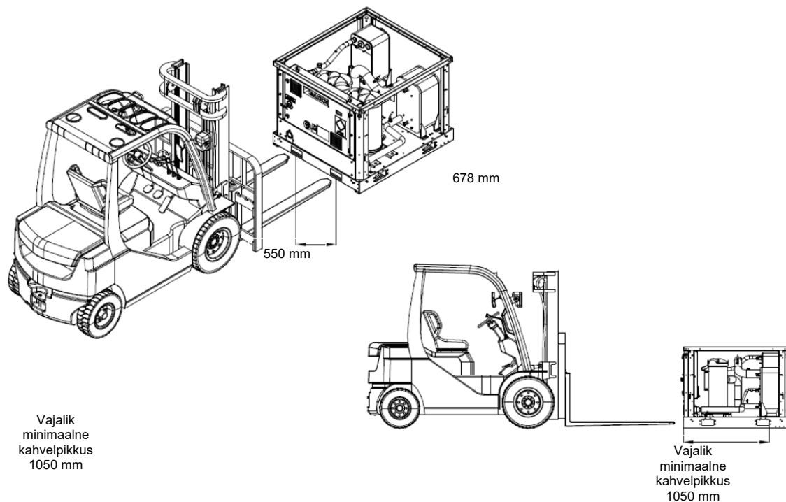
Joonis. 9 – Alternatiivne käsitlemisviis kahveltõstukiga
