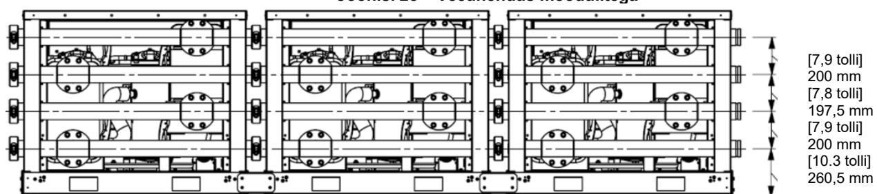
Joonis. 28 – Veeühendus moodulitega
