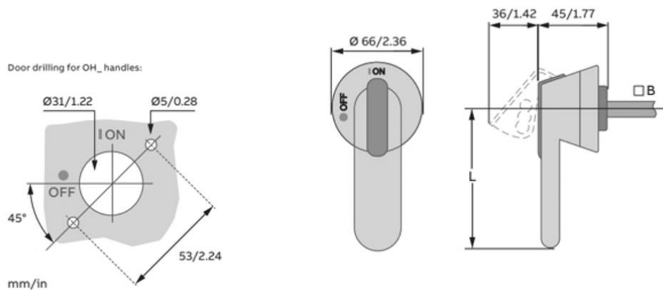
Joonis. 21 – Püstoli käepideme andmed
