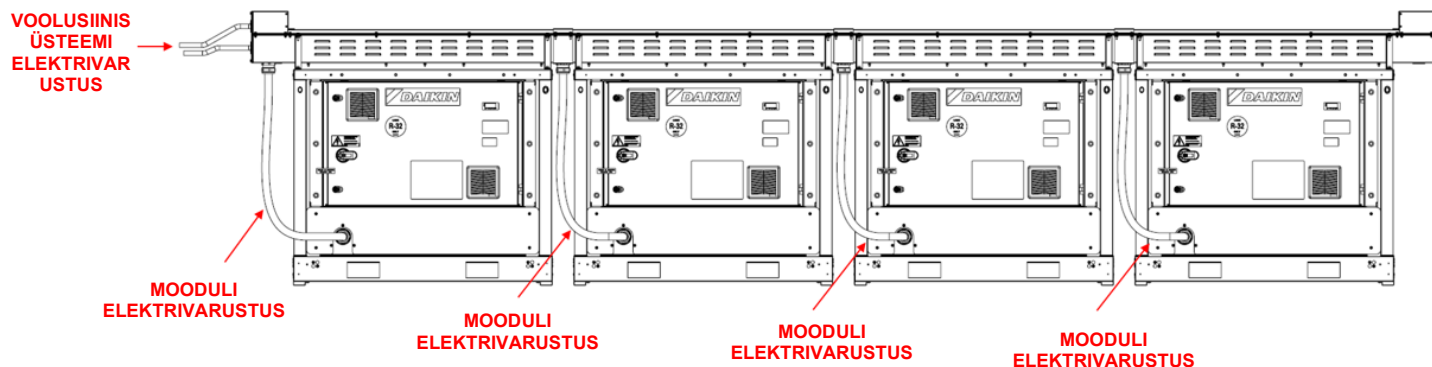
Joonis. 50 – Kaablite juhtimine latisüsteemi ja seadme vahel
