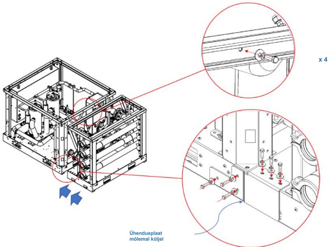
Joonis. 23 – Jahuti ja kollektori moodulite ühendamisjuhised
