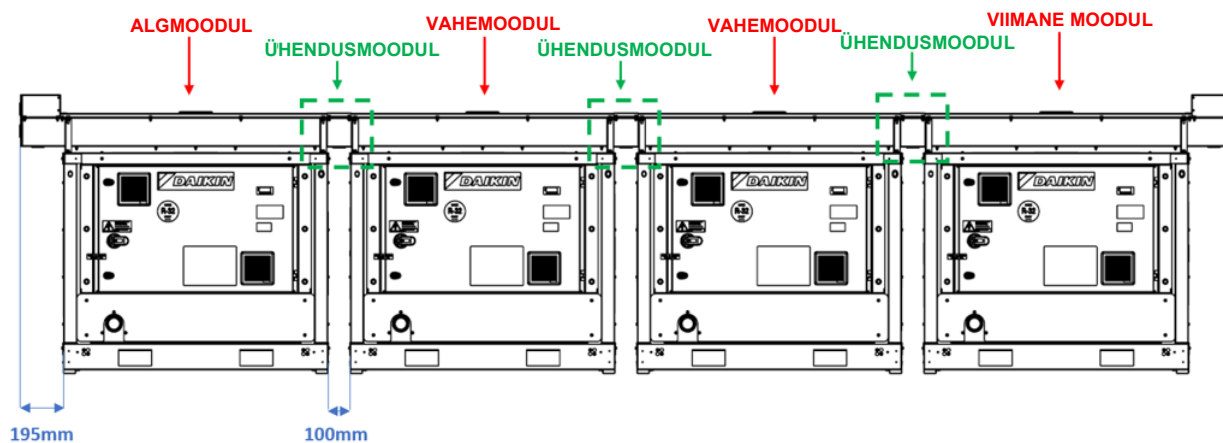
Joonis. 50 – Kaablite juhtimine latisüsteemi ja seadme vahel
