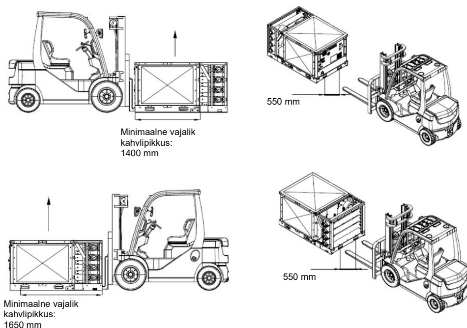
Joonis. 45 – Seadme ja kollektori moodulite käsitlemine
