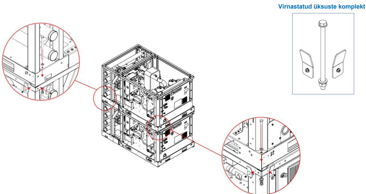
Joonis. 40 – Virnastatud üksuste paigaldusjuhised
