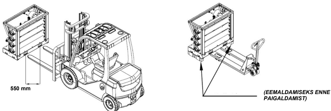
Joonis. 44 – Kollektormooduli käsitlemine
