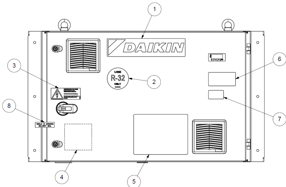
Joonis. 22 – Elektripaneelile kinnitatud siltide identifitseerimine (Standard*)
