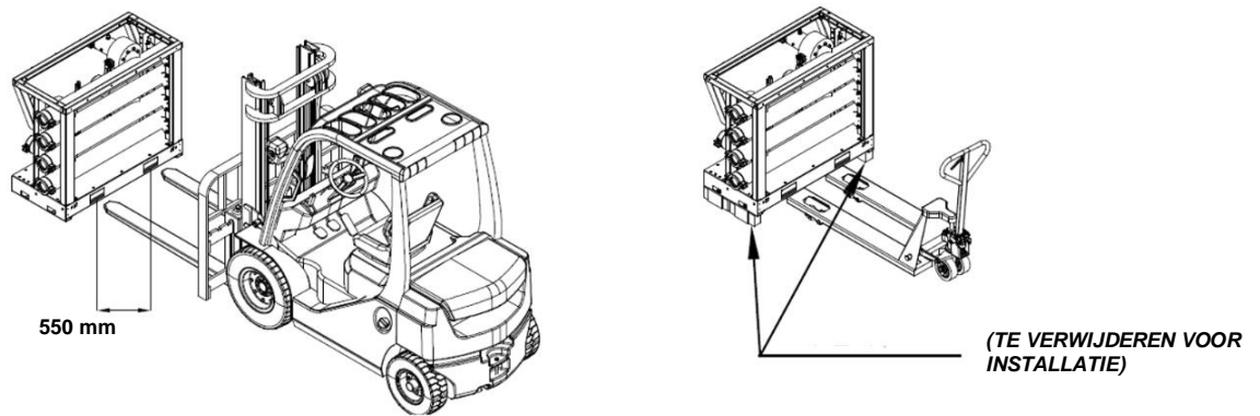
Fig. 44 - Behandeling van verdeelstukmodule
