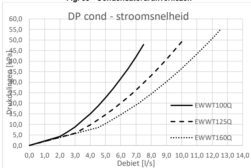
Fig. 63 - Condensatordrukverliezen
