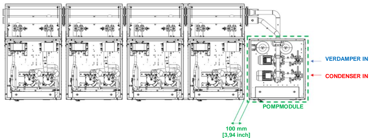
Fig. 43 - Installatie pompmodule - leidingdetails
