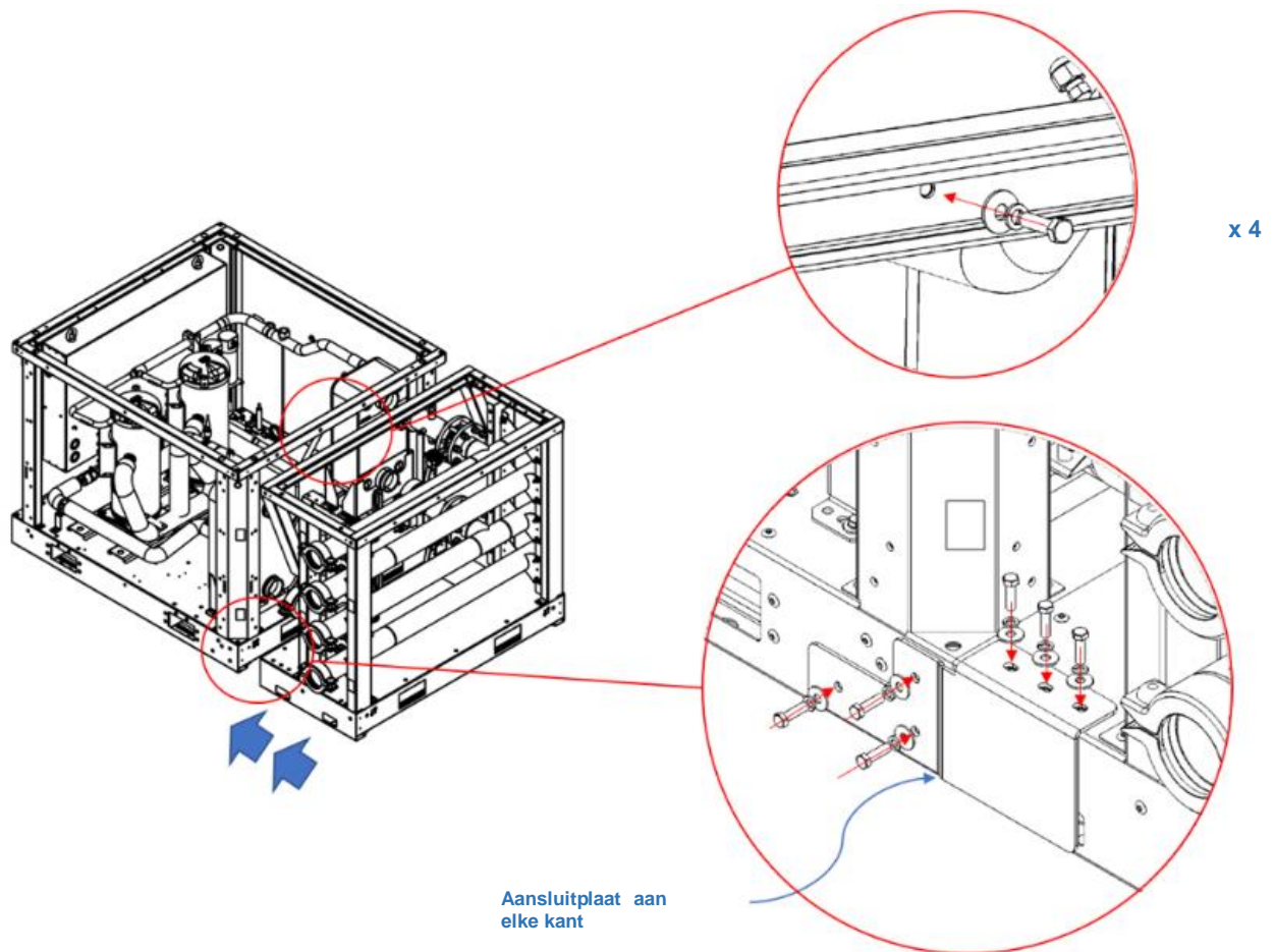
Fig. 23 - Aansluitinstructies tussen koelmachine en verdeelmodules
