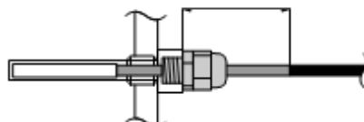
Fig. 16 - Watertemperatuursonde ≤50 mm
