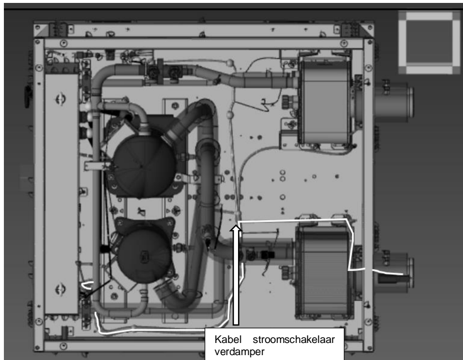
Fig. 13 - Kabels van de stroomschakelaar van de verdamper
