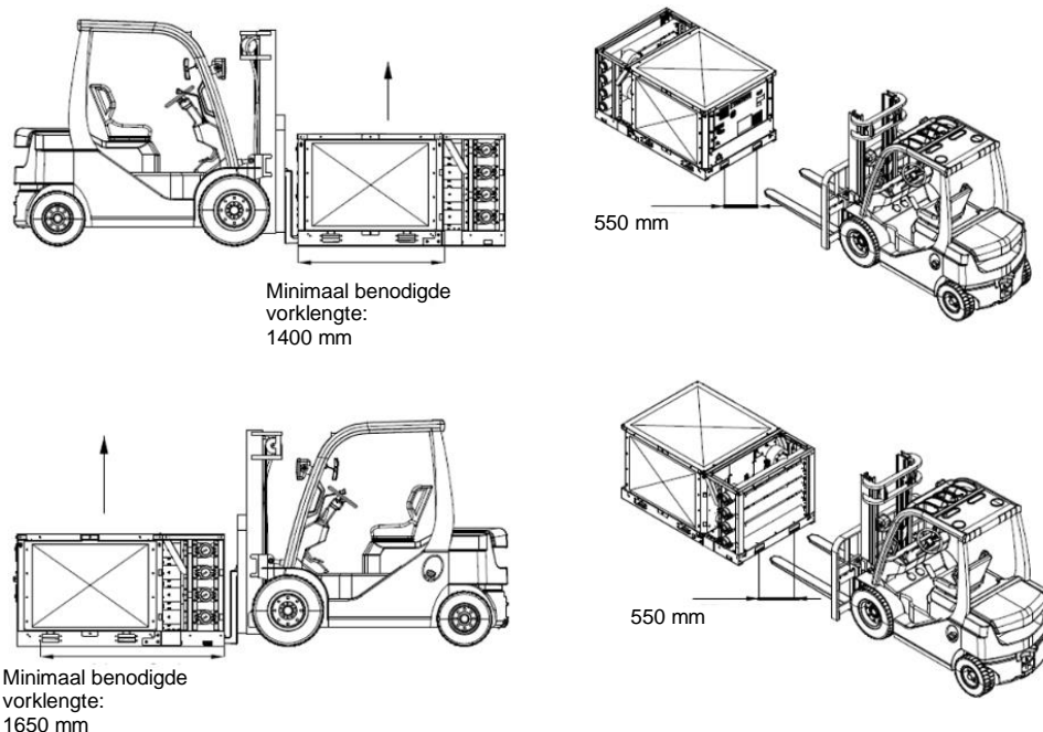
Fig. 45 - Behandeling van unit- en verdeelmodules
