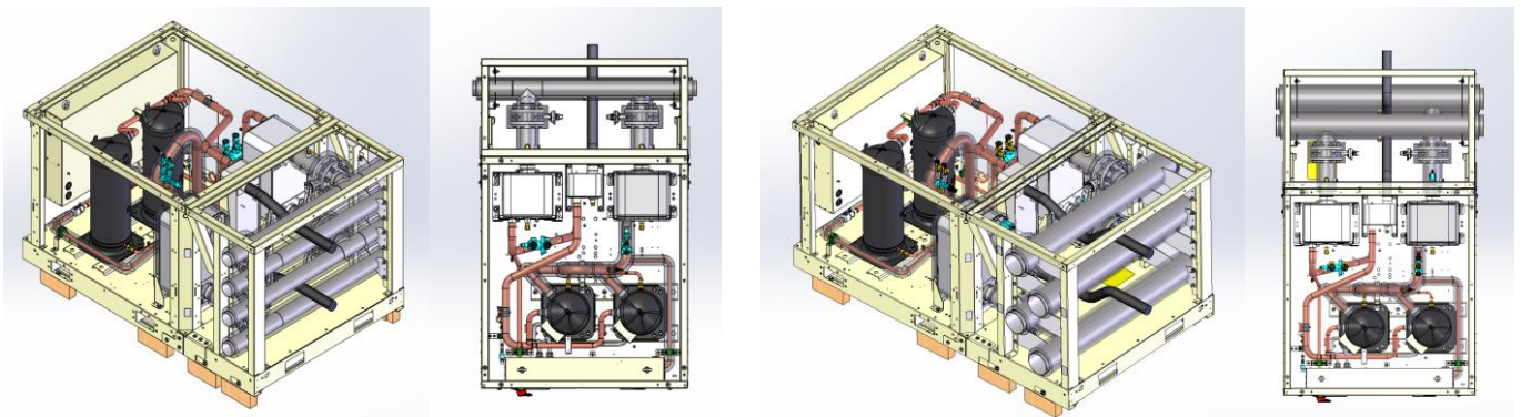
Fig. 24 - PHR-buizen met verdeelmodule (links voor 3inch - rechts voor 5inch-verdeelbuizen)
