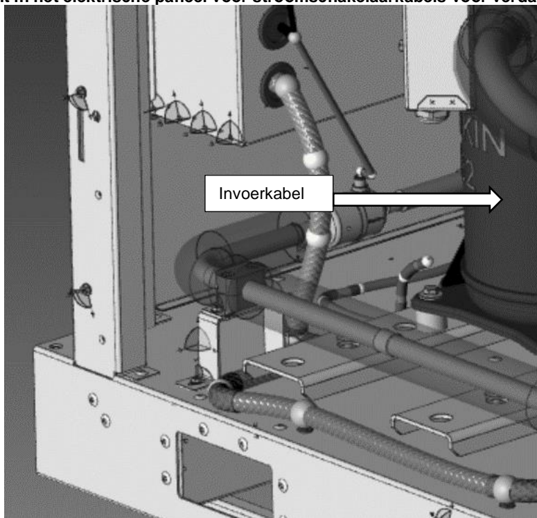
Fig. 15 - Invoerpunt in het elektrische paneel voor stroomschakelaarkabels voor verdamper en condensor
