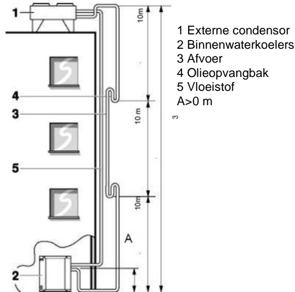
Fig. 17 - Koelmiddelcircuit aansluiten (1)
