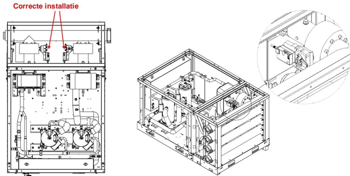
Fig. 31 - Montage-indicaties voor klepaandrijving
