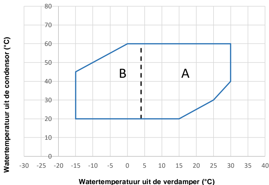
Fig. 7 - EWLT-Q Bedrijfslimieten
