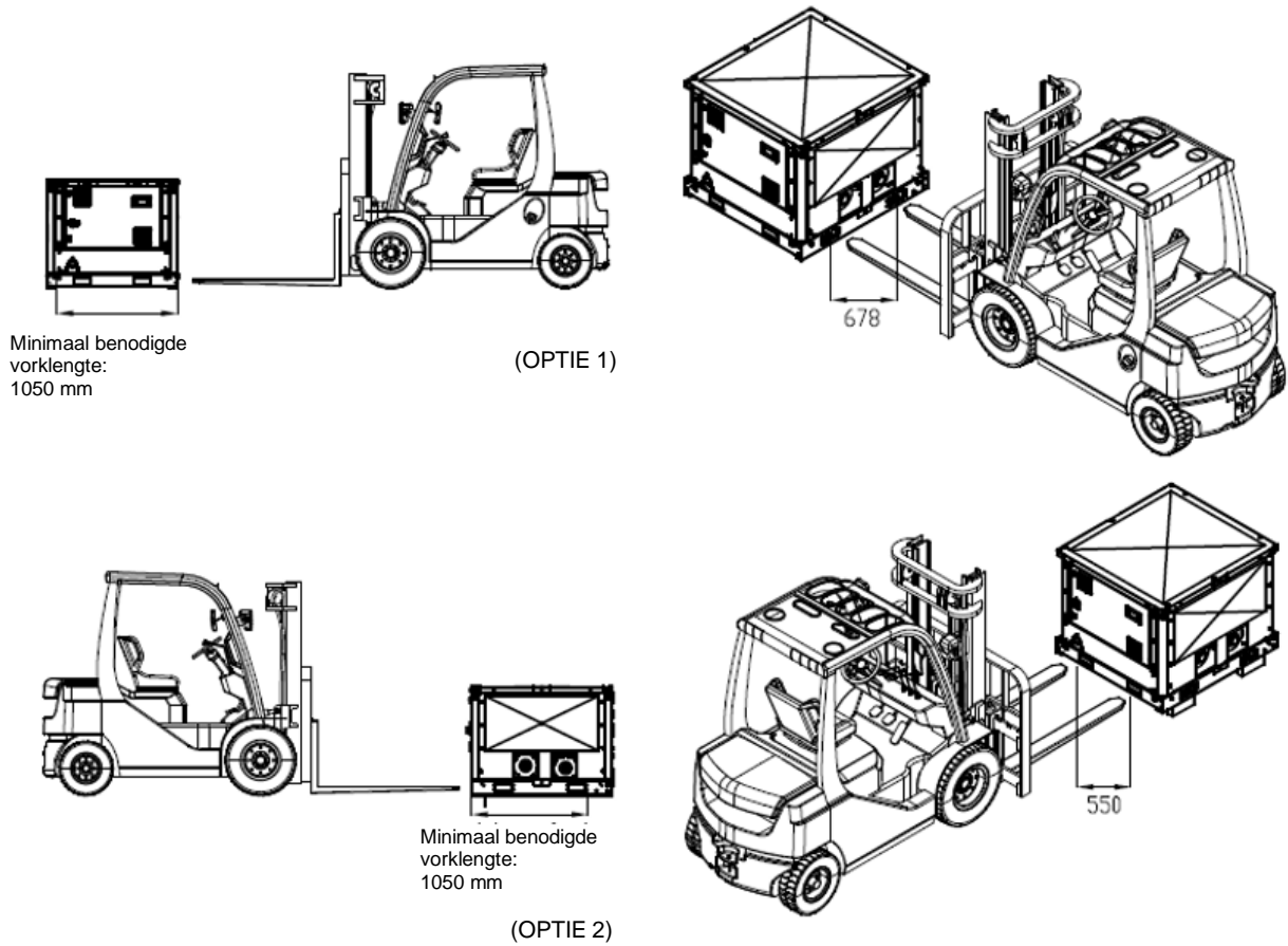
Fig. 47 - Hantering van pompmodule met vorkheftruck
