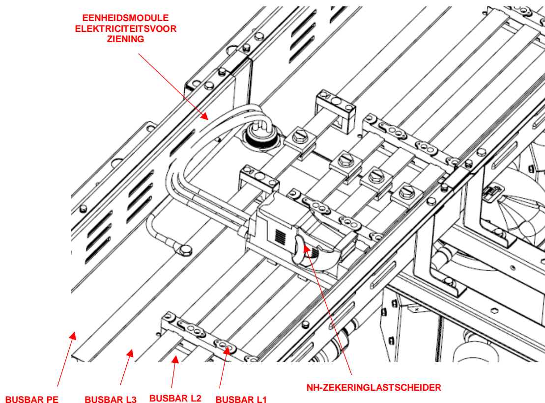
Fig. 57 - Detail van de elektrische aansluiting voor een andere unitmodule
