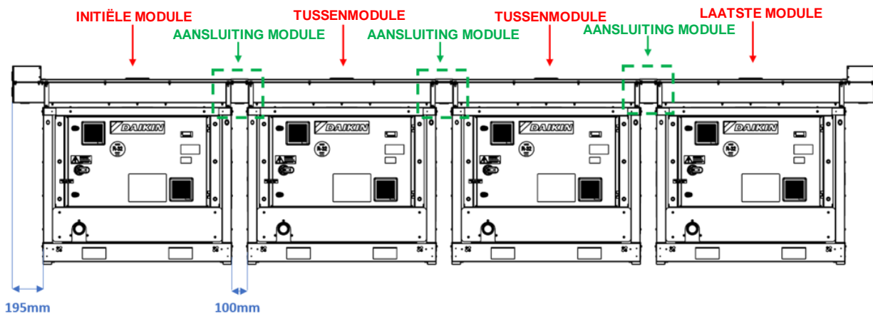
Fig. 50 - Kabeldoorvoer tussen barsysteem en unit
