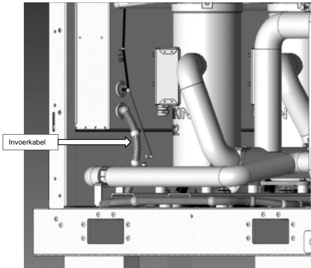
Fig. 38 - Elektrische paneelingang voor bedieningskabels voor verdamper- en condensorafsluitkleppen
