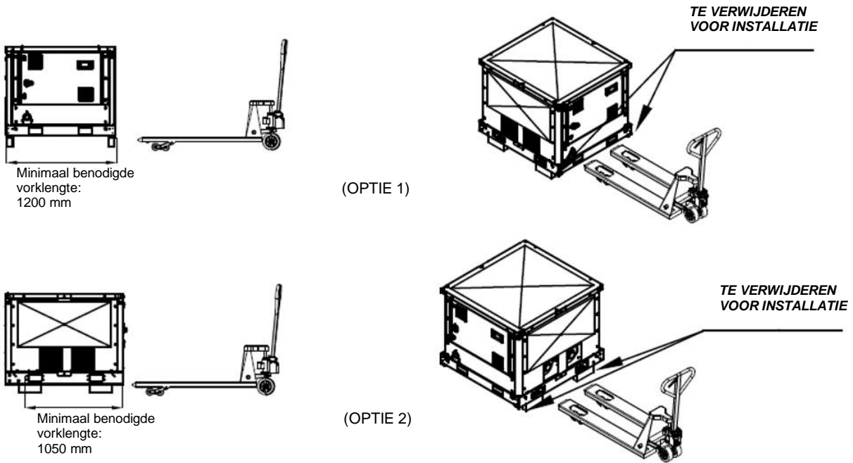
Fig. 48 - Behandeling van pompmodule met behulp van pallettruck
