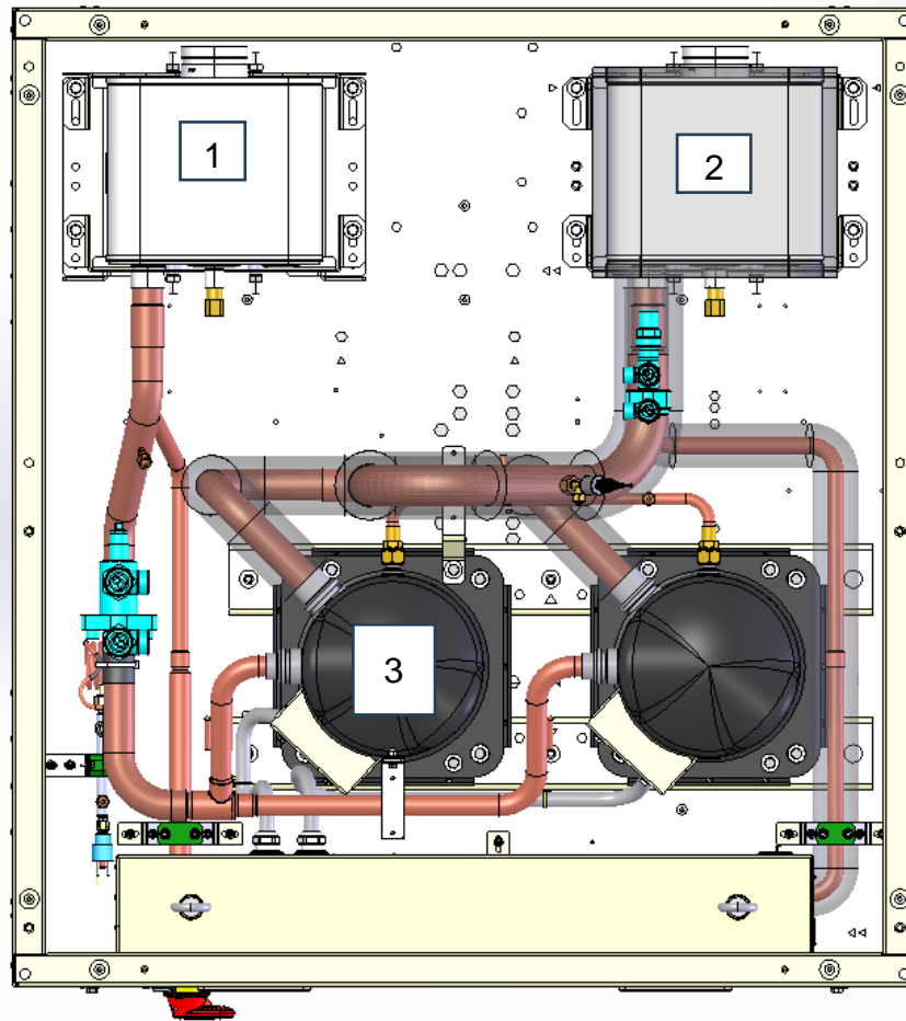
Fig. 11 - Referentietekening voor identificatie van verdamper en condensor
