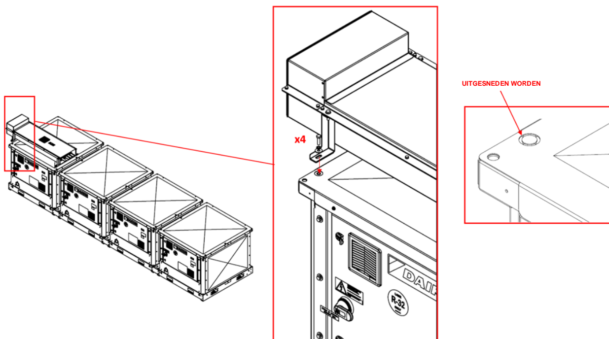
Fig. 52 - Bevestiging van het stroomrailsysteem aan de eenheid
