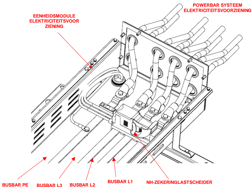
Fig. 56 - Detail van de elektrische aansluiting voor de module van de eerste eenheid
