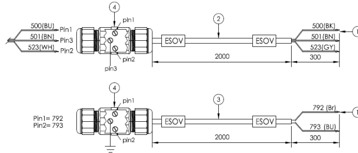
Fig. 34 - Kabeladapters voor condensorafsluitklepactuator en eindschakelaars
