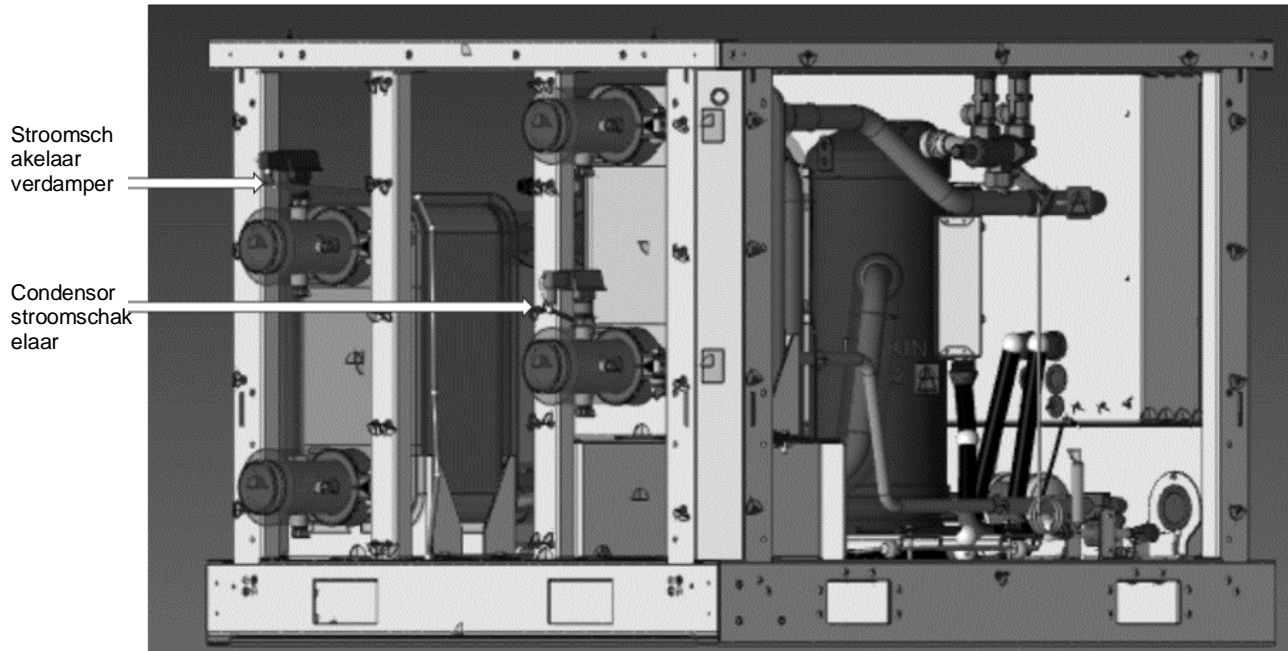
Fig. 13 - Kabels van de stroomschakelaar van de verdamper
