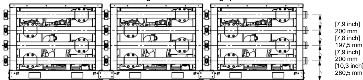
Fig. 28 - Wateraansluiting op modules
