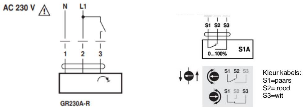
Fig. 32 - Aansluitschema voor motor (linker figuur) en eindschakelaars (rechter figuur)
