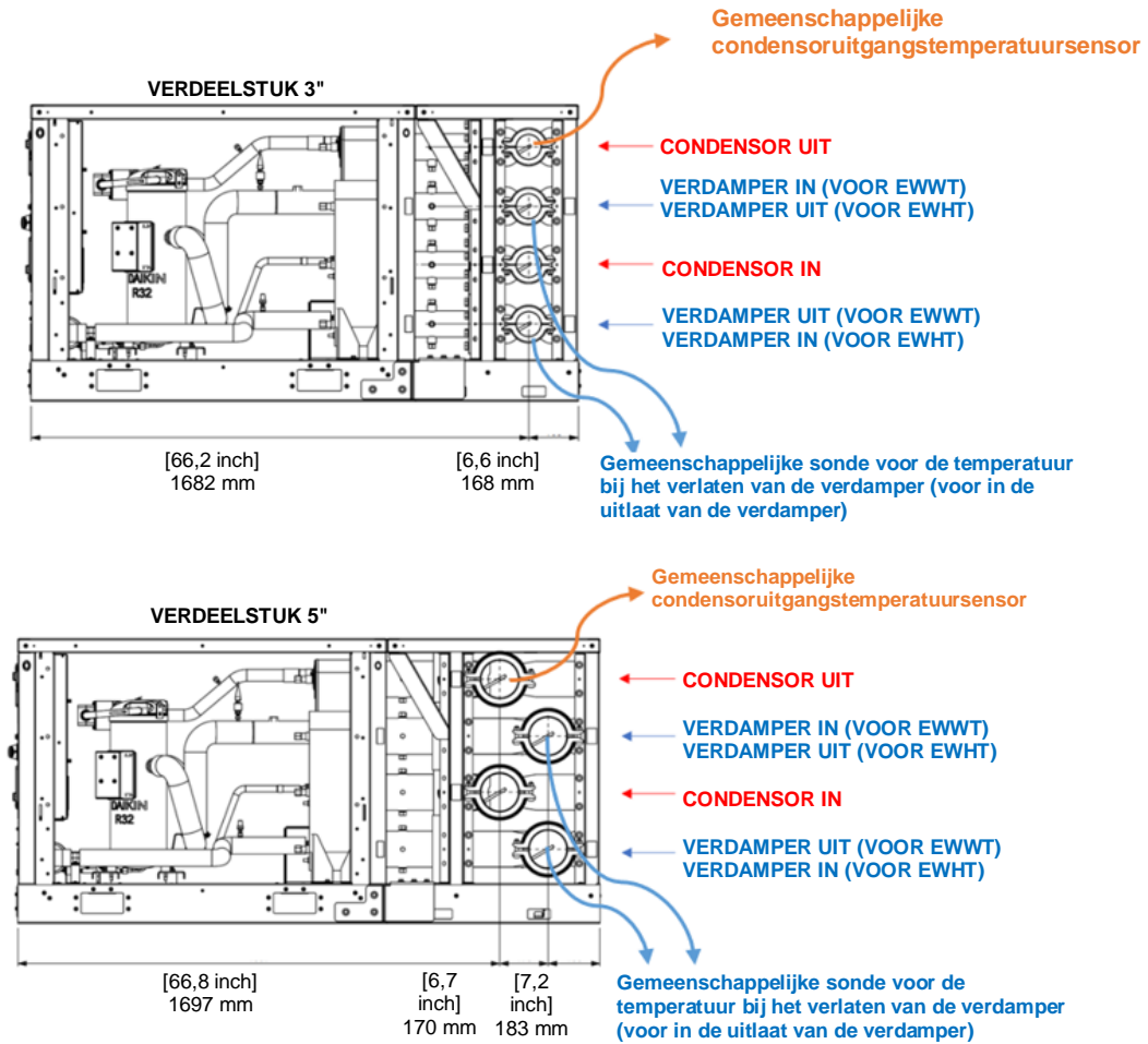
Fig. 59 - Posities van de temperatuursensoren voor 3" en 5" verdeler
