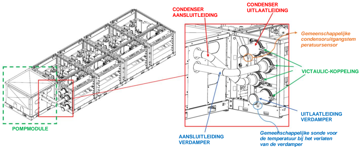
Fig. 60 - Details van de plaatsing van de sondes op de pijpen
