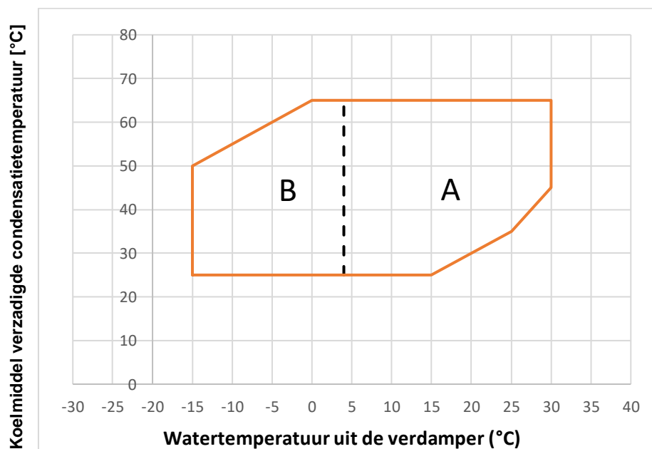
Fig. 7 - EWLT-Q Bedrijfslimieten
