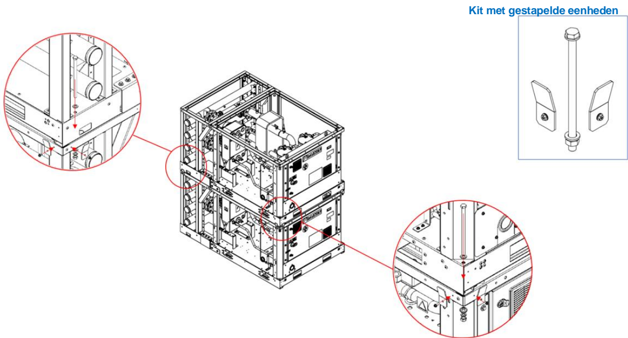
Fig. 40 - Montage-instructies voor gestapelde eenheden
