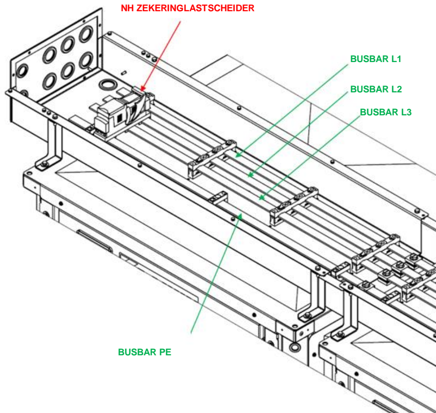
Fig. 55 - Detail van de zekeringen en van de doos voor kabeldoorvoer van de voedingsbalkmodule
