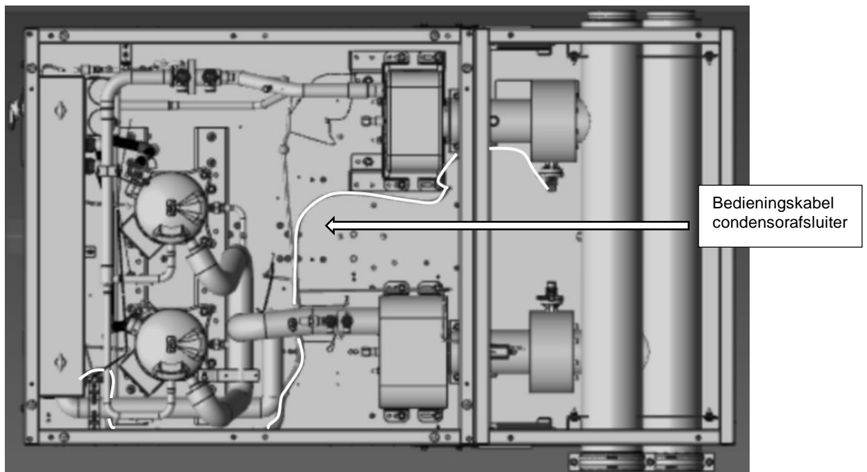
Fig. 37 - Kabelgeleiding van de condensatorafsluiter
