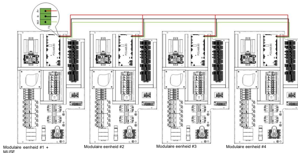
Fig. 61 - Aansluiting van 4 PLC's op hetzelfde Modbus-netwerk
