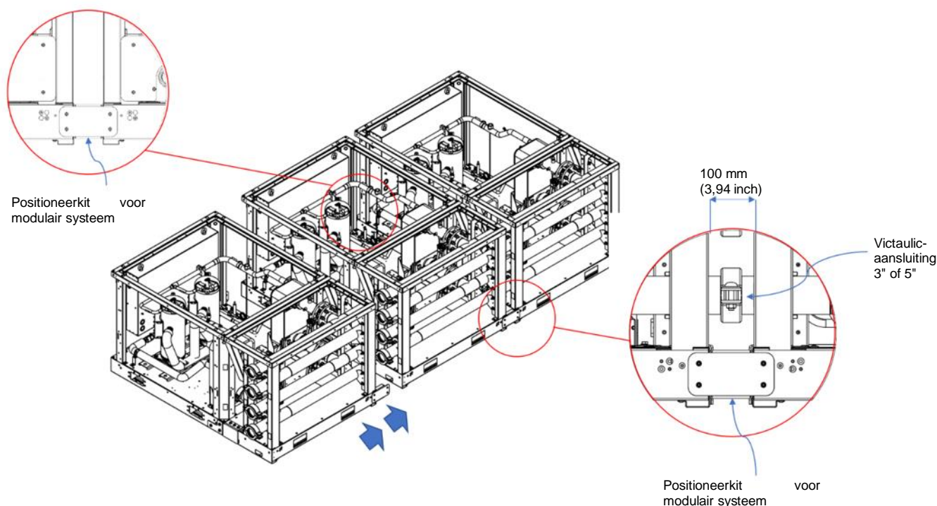
Fig. 26 - Aansluiting modulaire systemen
