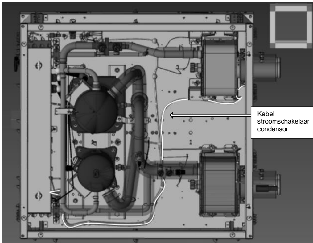
Fig. 15 - Invoerpunt in het elektrische paneel voor stroomschakelaarkabels voor verdamper en condensor
