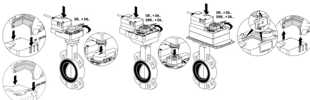
Fig. 30 - Montage-instructies voor aandrijver-eindschakelaars
