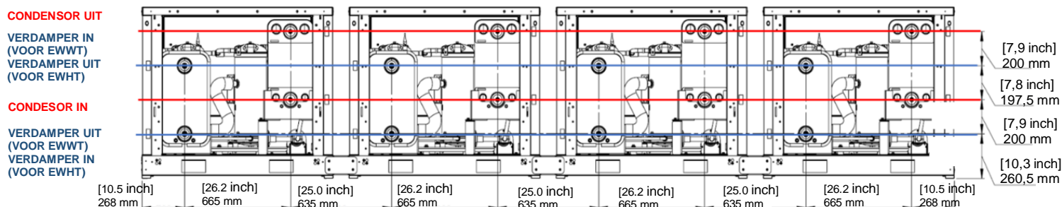
Fig. 25 - Waterleidingconfiguratie
