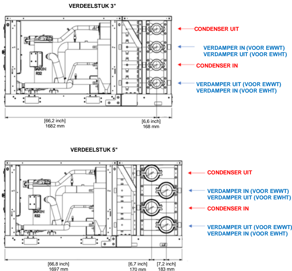
Fig. 27 - Afmetingen waterverdeler
