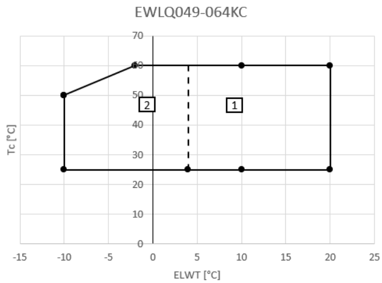
Εικόνα 4 - EWLQ049-064KC
