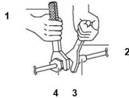
Εικόνα 6 - Σύνδεση του κυκλώματος ψυκτικού μέσου (2)
