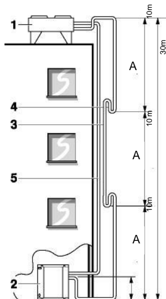
Obrázek 5- Připojení okruhu chladiva (1).
