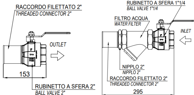
Rysunek 16 – Elementy hydrauliczne
