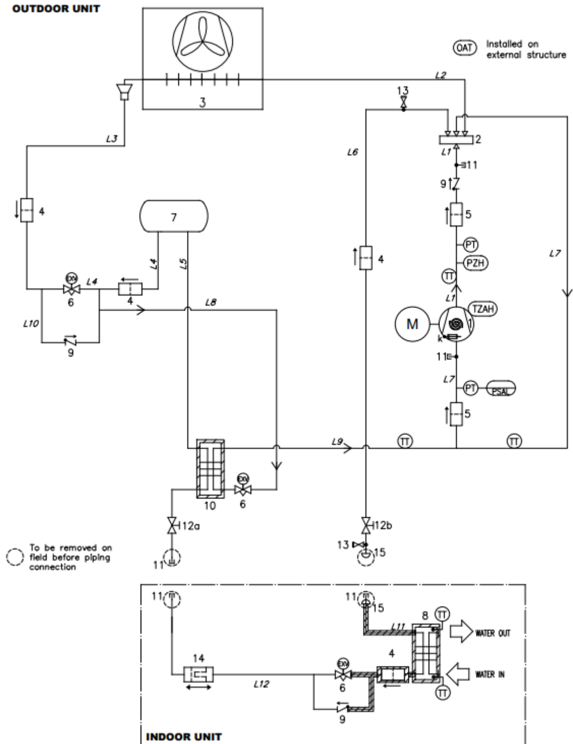
23. ábra – Hűtőközeg-kör (P&ID) diagramja MONO körnél EWT-CZ egységen
