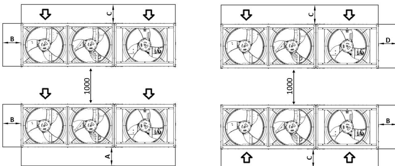
Figure 11 – Unités installées côte à côte le long de leurs côtés les plus longs (cas 1 et cas 2)
