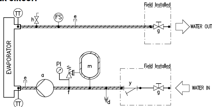
Εικόνα 15 – Υδραυλικό διάγραμμα
