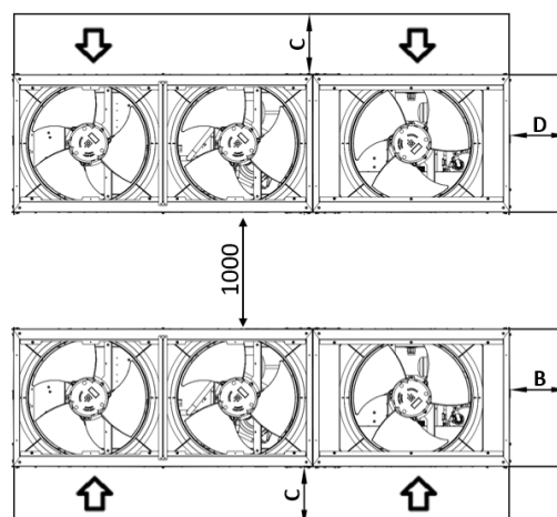
Εικόνα 11 – Μονάδες εγκατεστημένες η μία δίπλα στην άλλη κατά μήκος των μεγαλύτερων πλευρών τους (Περίπτωση 1 και Περίπτωση 2)
