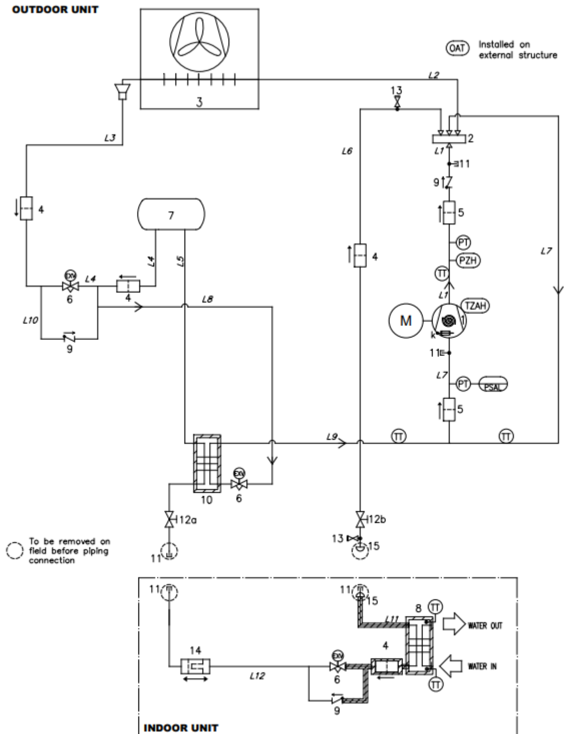
Εικόνα 23 – Διάγραμμα κυκλώματος ψυκτικού μέσου (P&ID) για μονάδα MONOY κυκλώματος EWT~CZ
